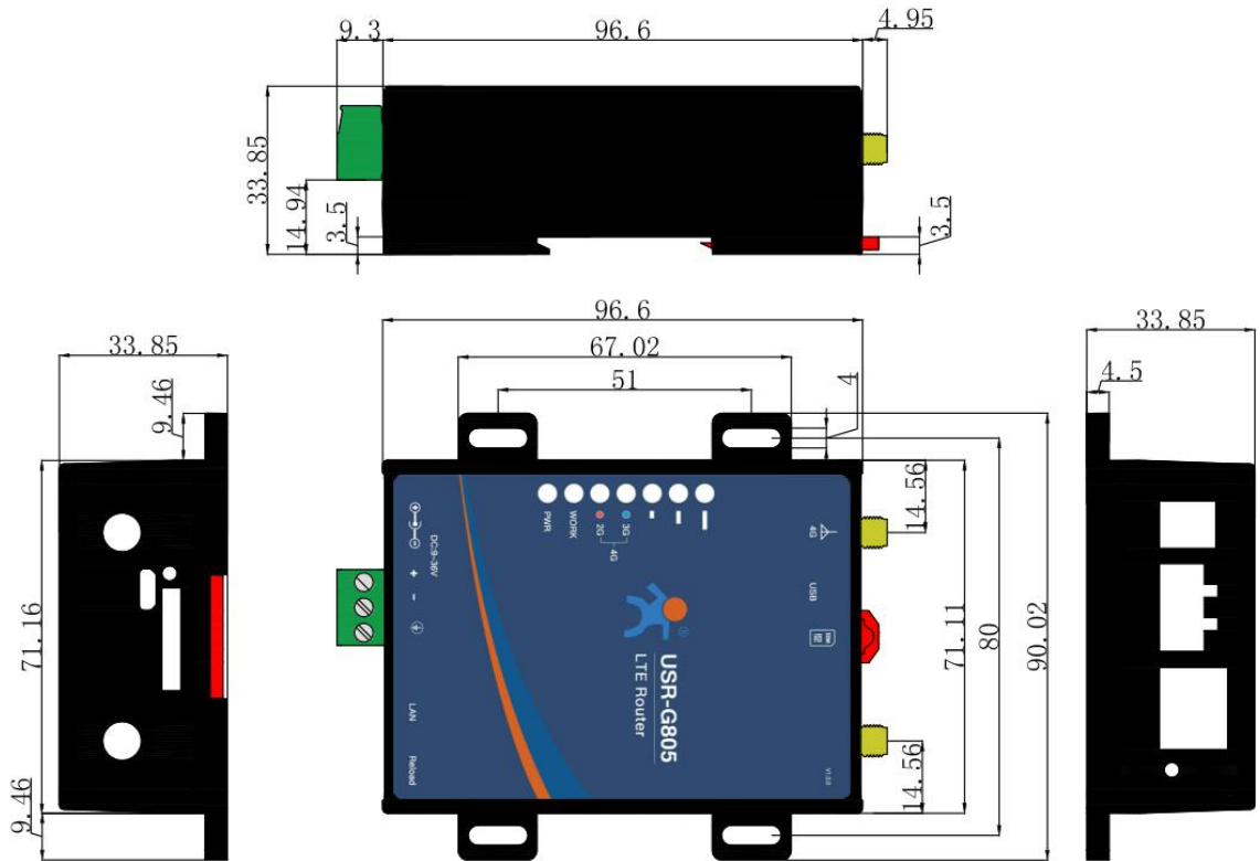
图 1 USR-G805 外观尺寸图
