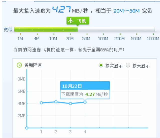
图 6 网络测速
