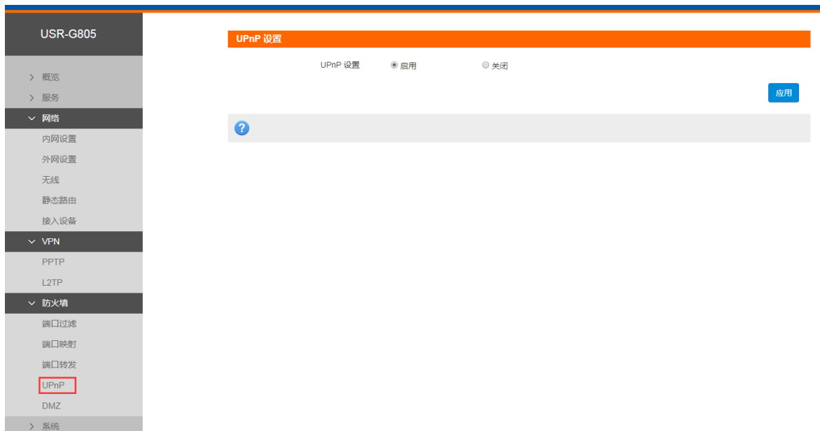
图 57 UPnP 页面
