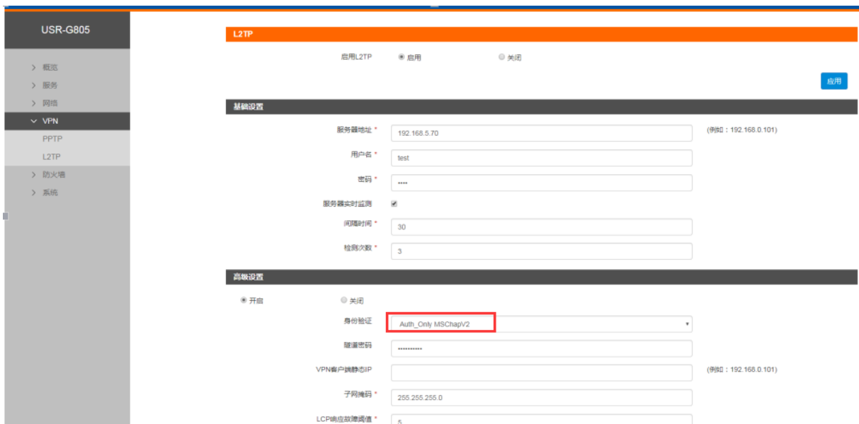
图 52 L2TP 基本设置
