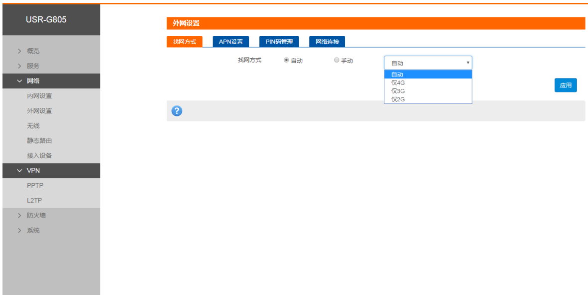
图 29 找网方式
