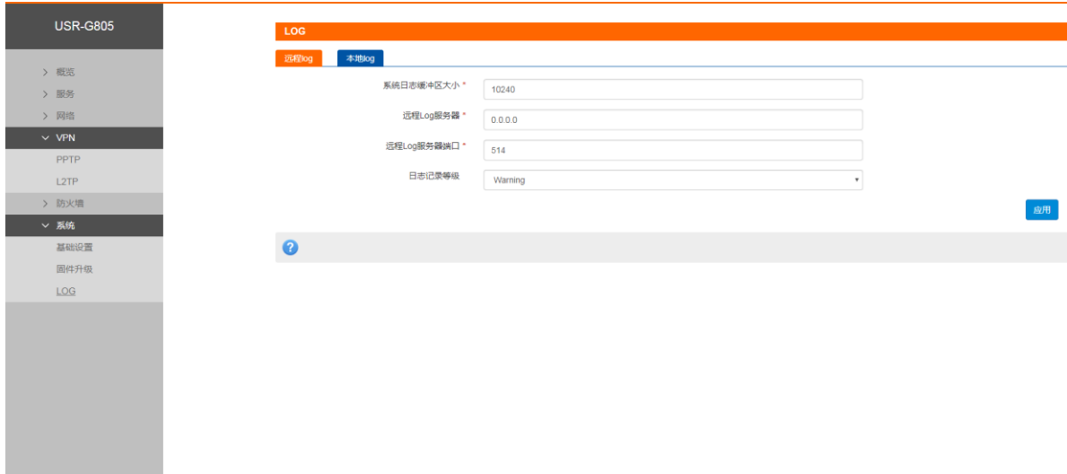
图 21 远程日志
