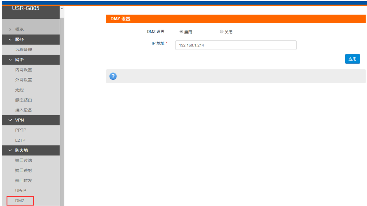
图 58 DMZ
