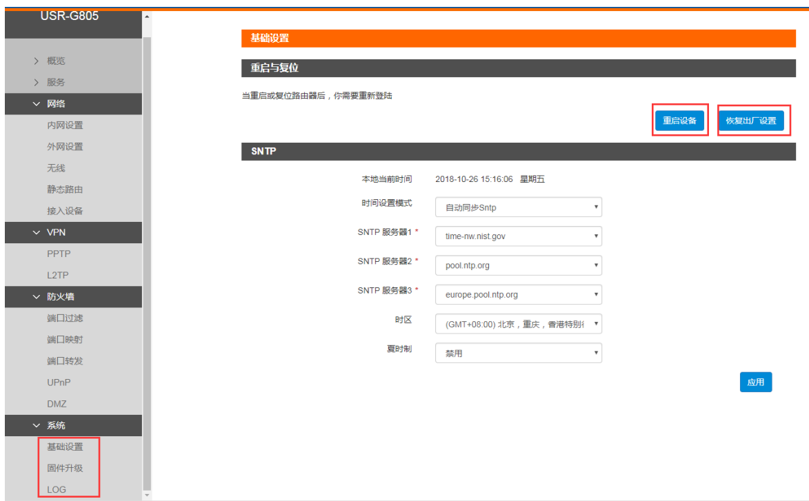
图 11 系统界面
