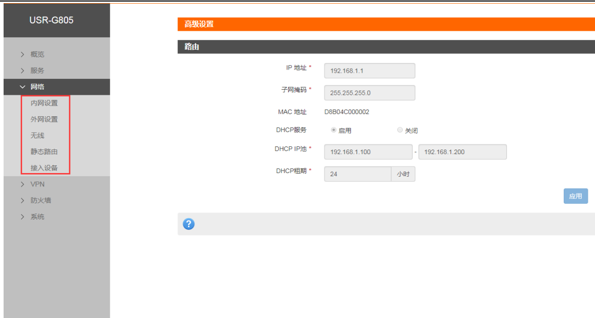
图 10 网络界面
