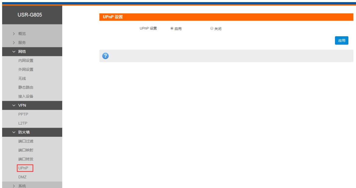
图 57 UPnP 页面
