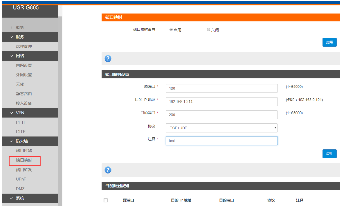
图 55 端口映射
