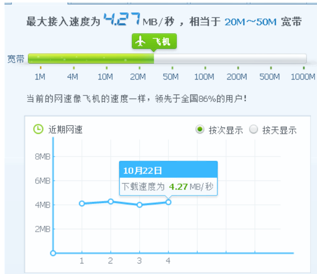
图 6 网络测速
