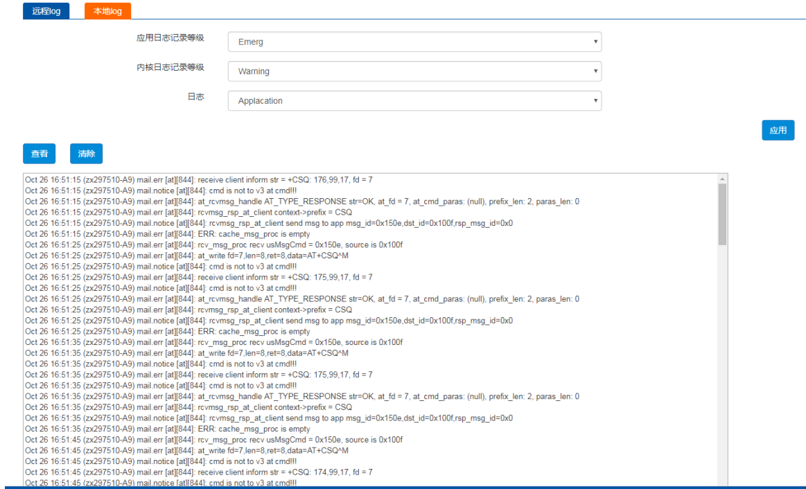
图 22 应用 log
