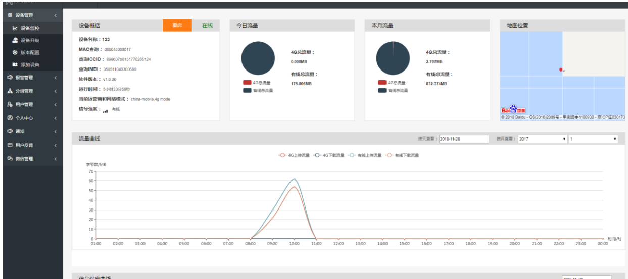
图 61 远程监控二
