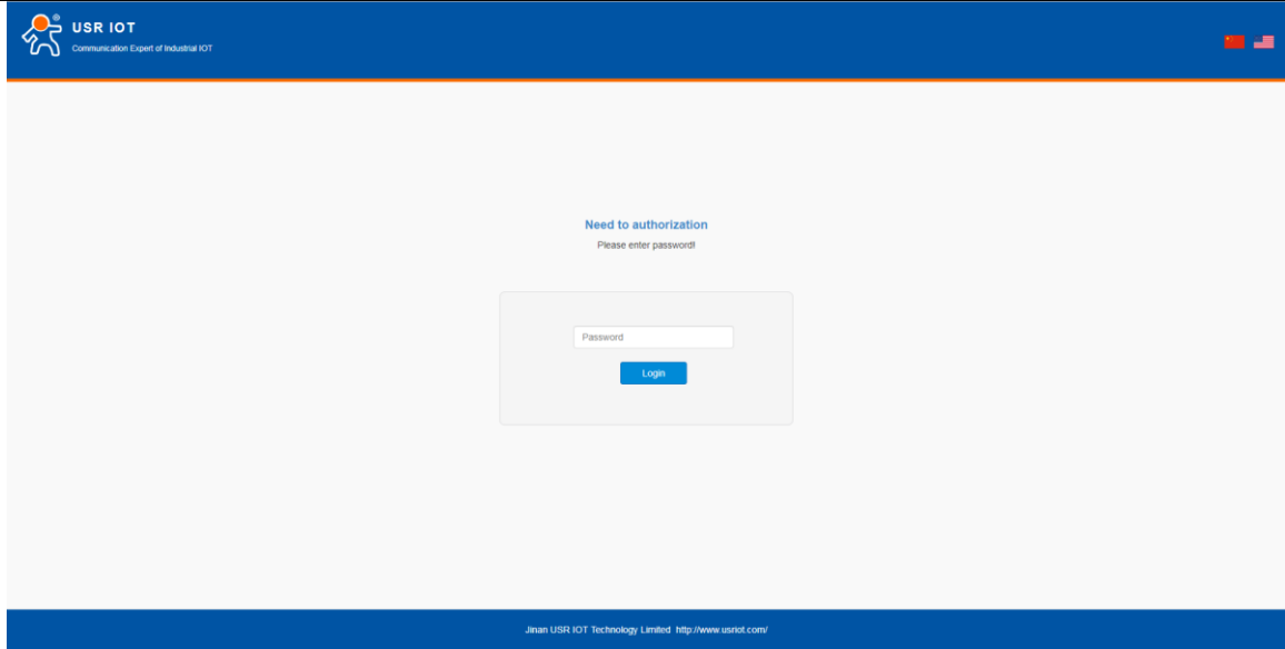
图 8 英文页面
