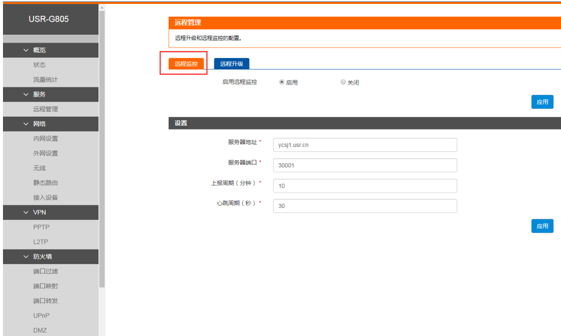
图 65 远程监控
