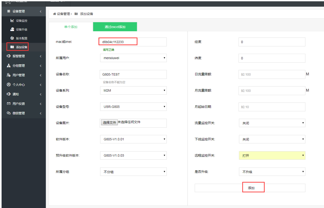
图 59 添加设备
