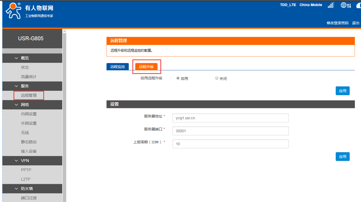
图 64 远程升级
