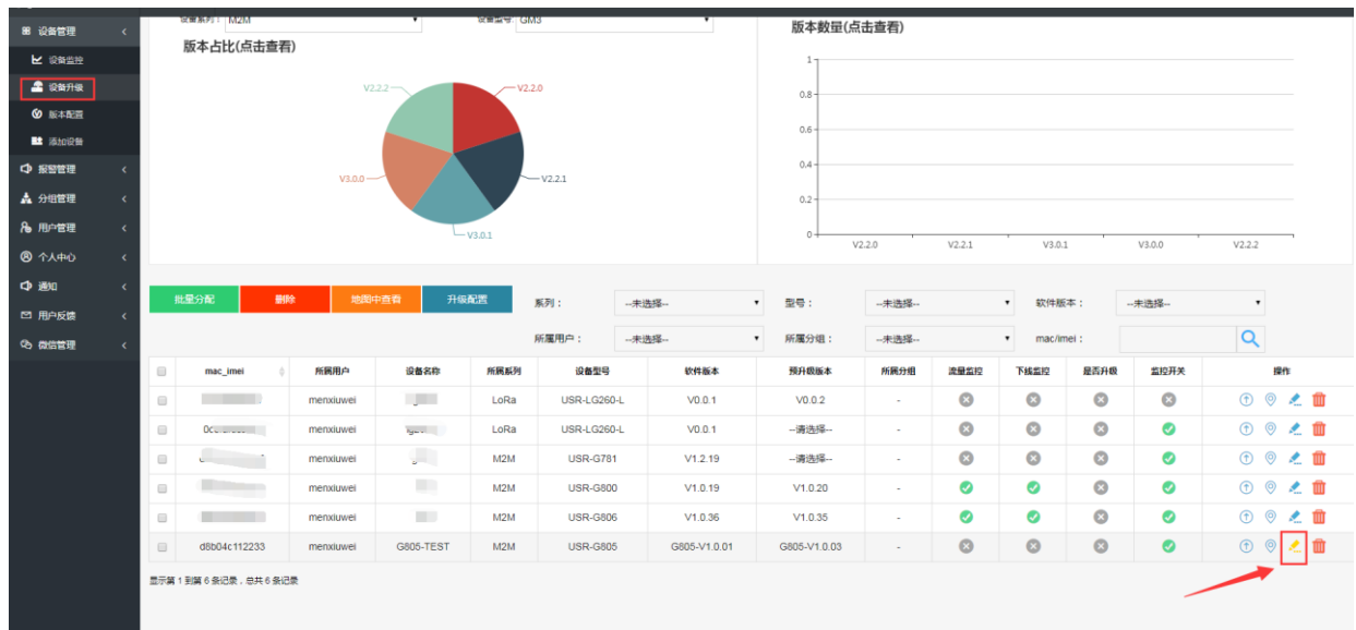
图 62 远程升级一
