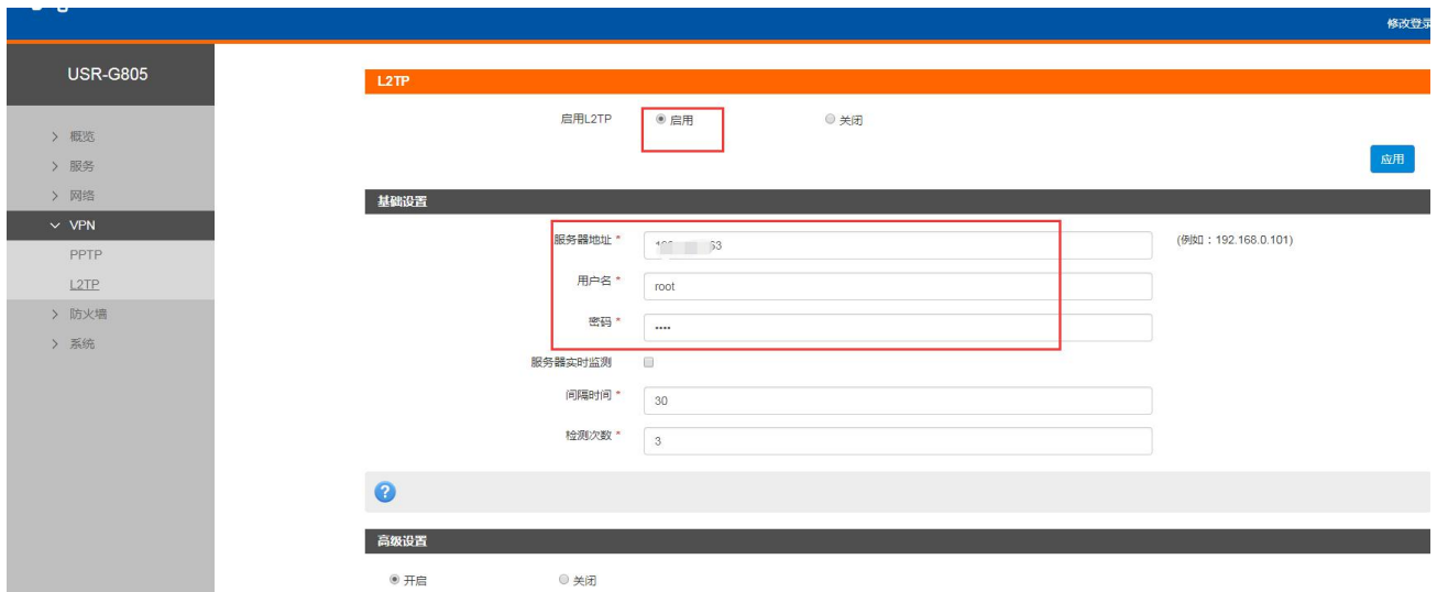
图 57 L2TP 搭建示例：基础设置
