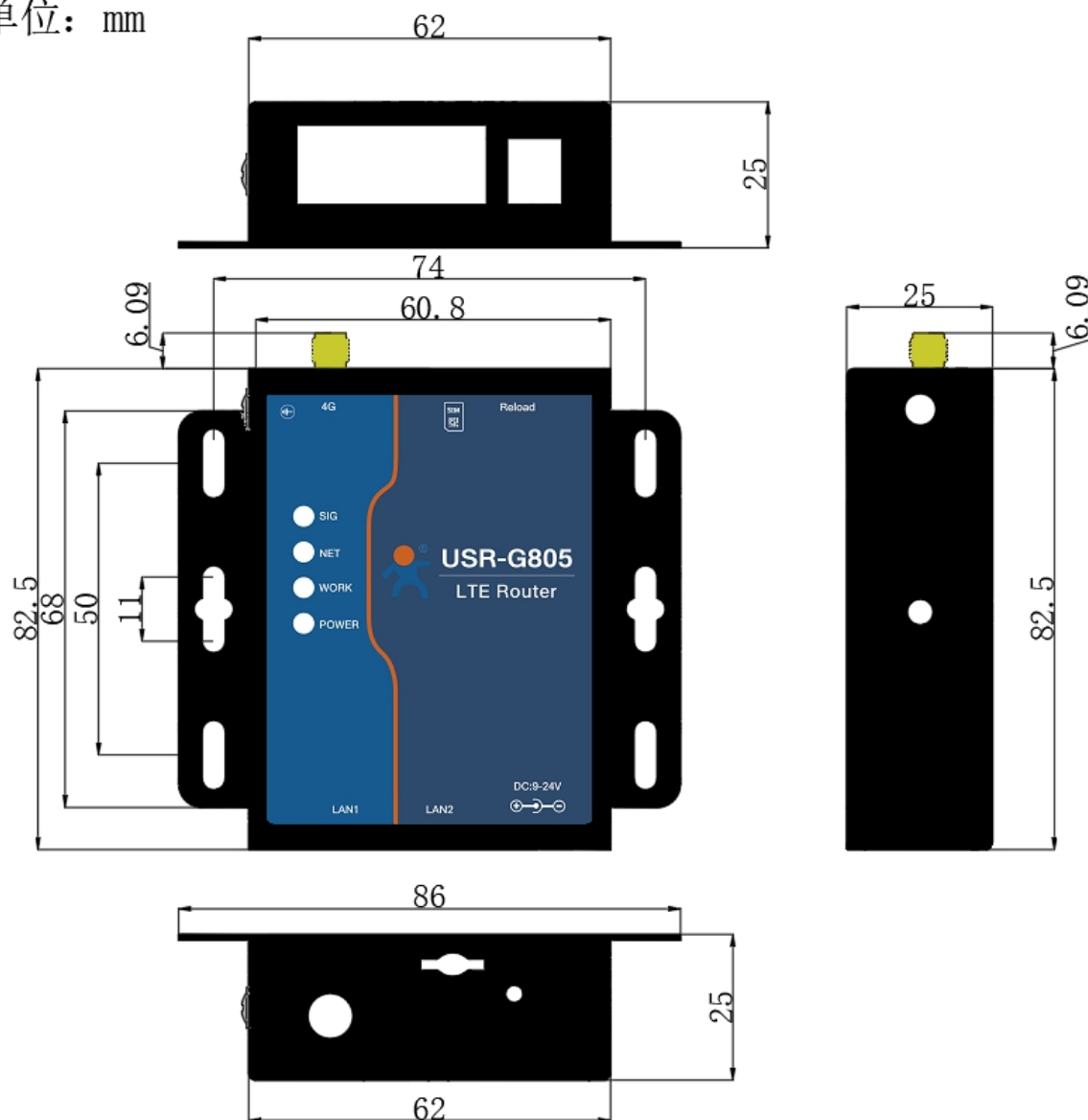
USR-G805c 产品尺寸
