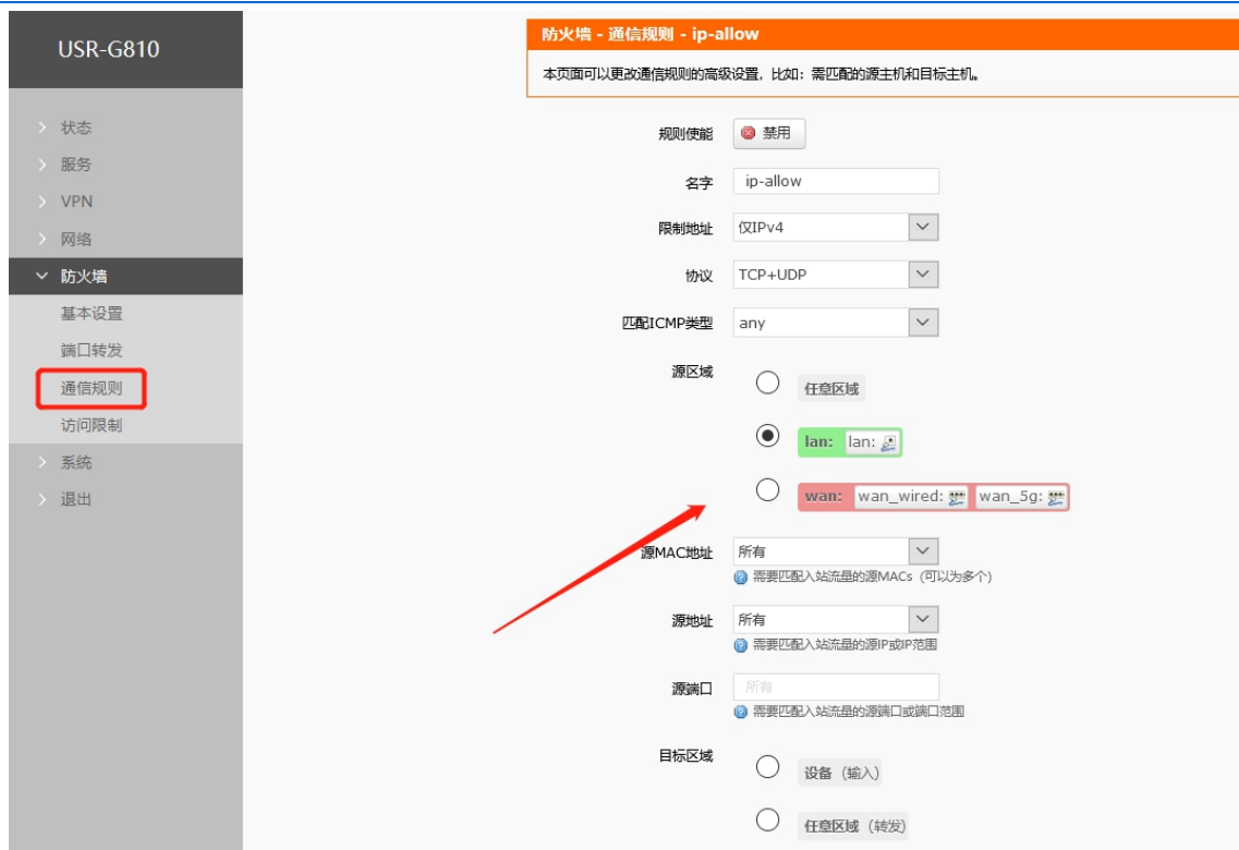
图 64 防火墙 IP 白名单图二
