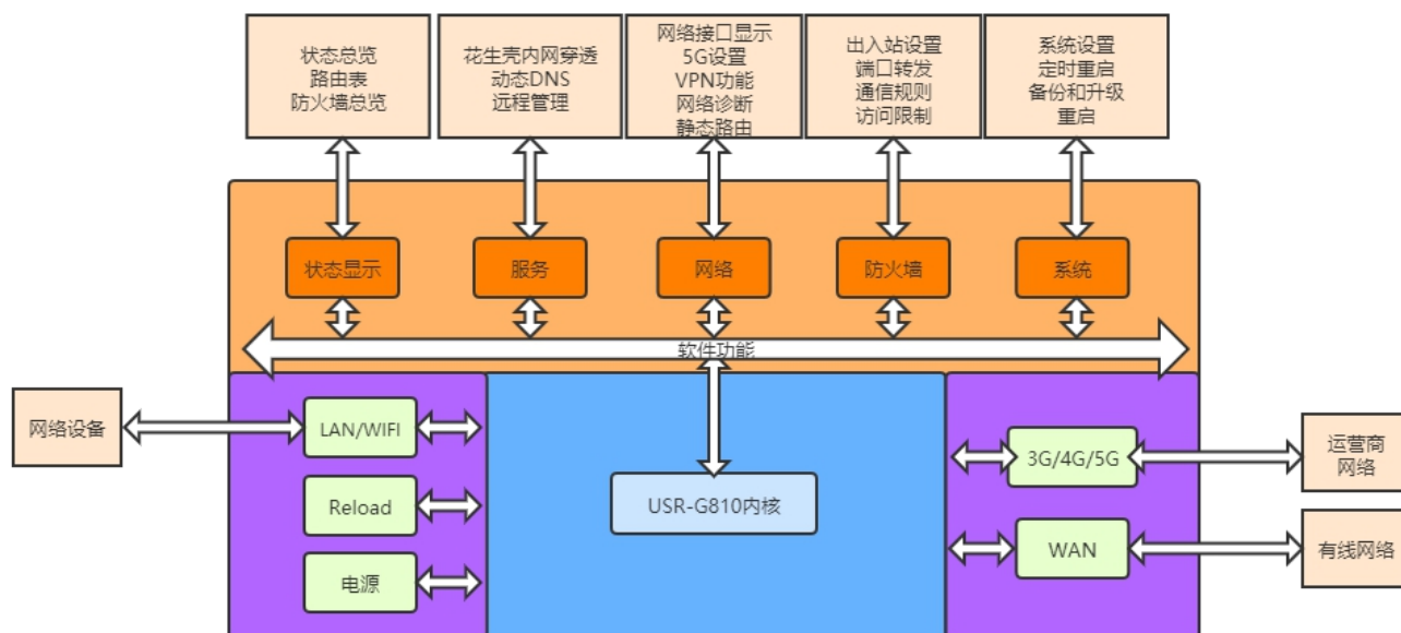
图 2 功能框图
