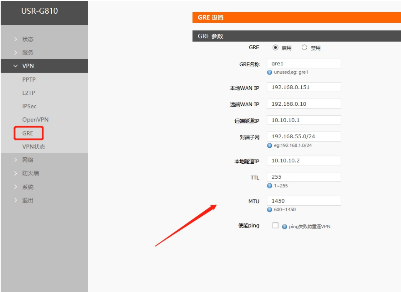
图 49 GRE 基本配置
