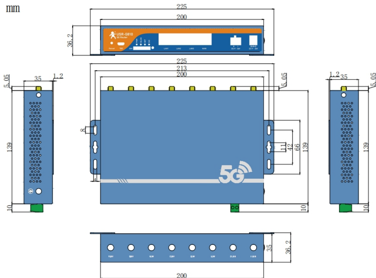
图 1 USR-G810 尺寸图
