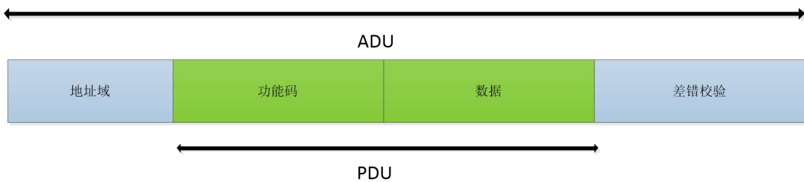
图 34 Modbus RTU 帧
