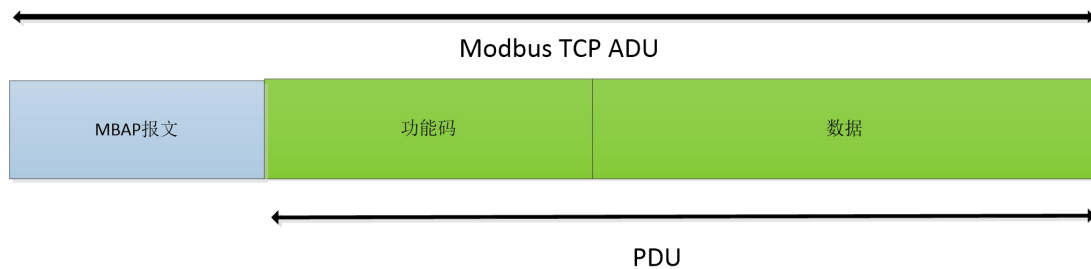
图 35 Modbus TCP 帧
