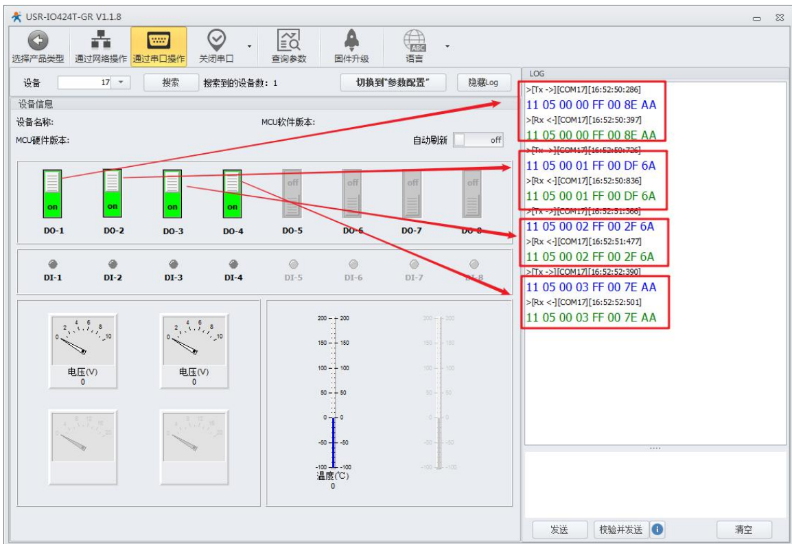
图 9 改变输出
