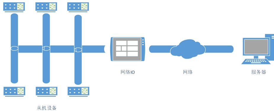
图 25 主机模式联网应用示意
