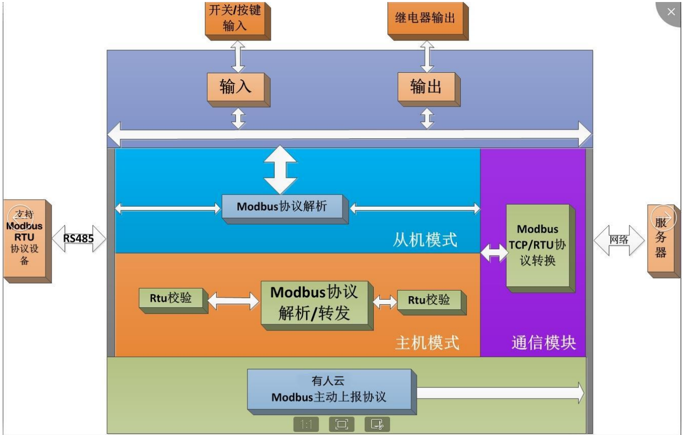
图 16 USR-IO424T-CAT1 功能框图
