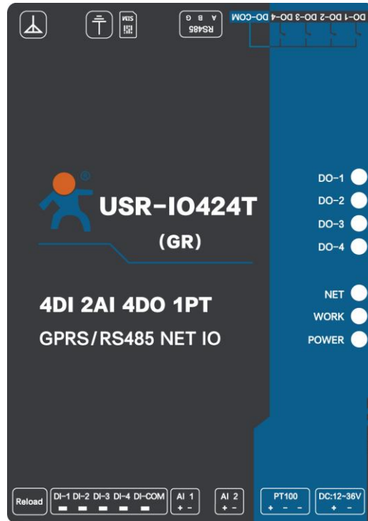
图 10 硬件接口示意图
