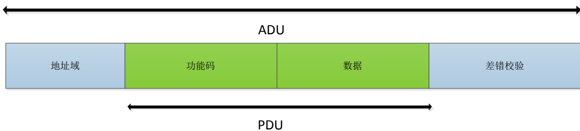
图 29 Modbus RTU 帧
