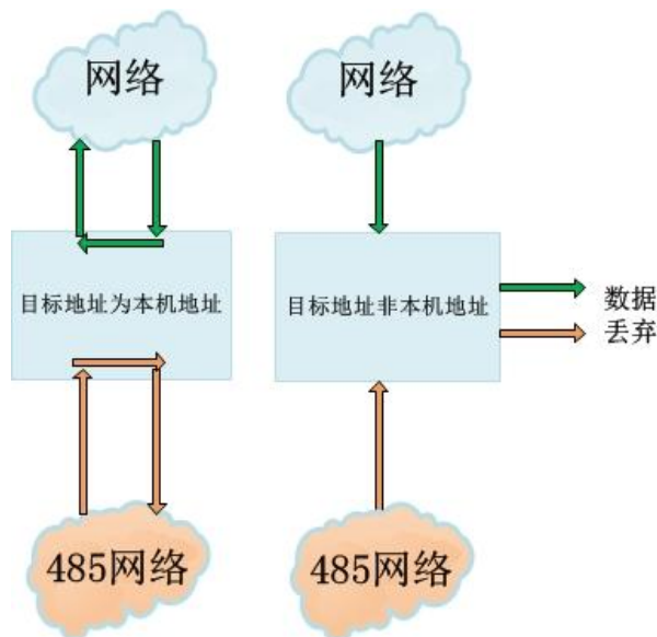
图 14 从机模式数据流向图
