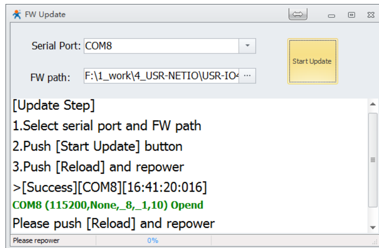
图 15 开始升级
