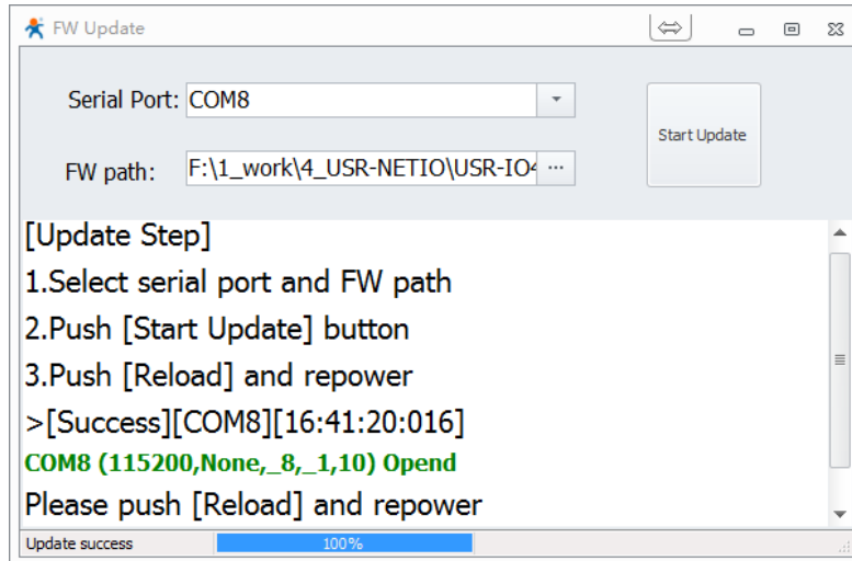
图 16 升级完成
