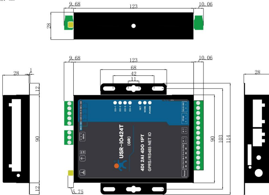
I0424-GR外观尺寸图
