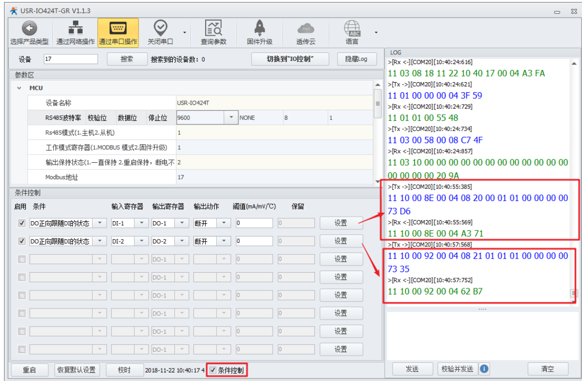
图 17 条件控制操作界面图
