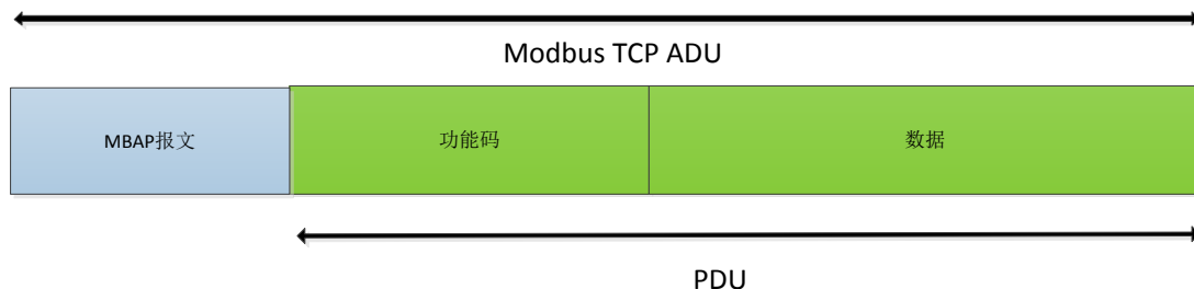
图 30 Modbus TCP 帧
