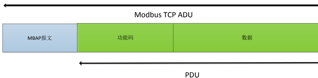
图 34 Modbus TCP 帧
