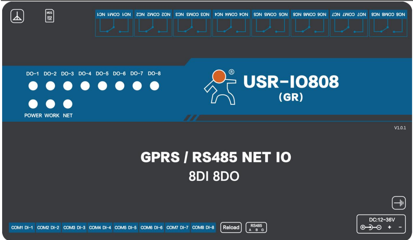
图 13 USR-IO808-GR V2 硬件接口示意图
