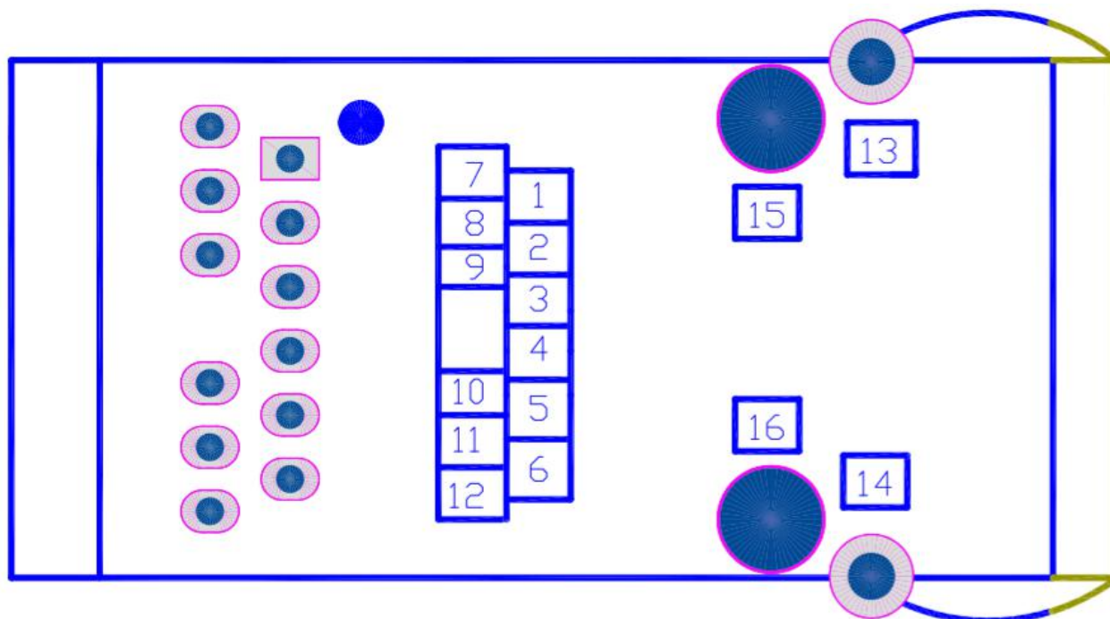
图 7 USR-K7 正视图引脚图
