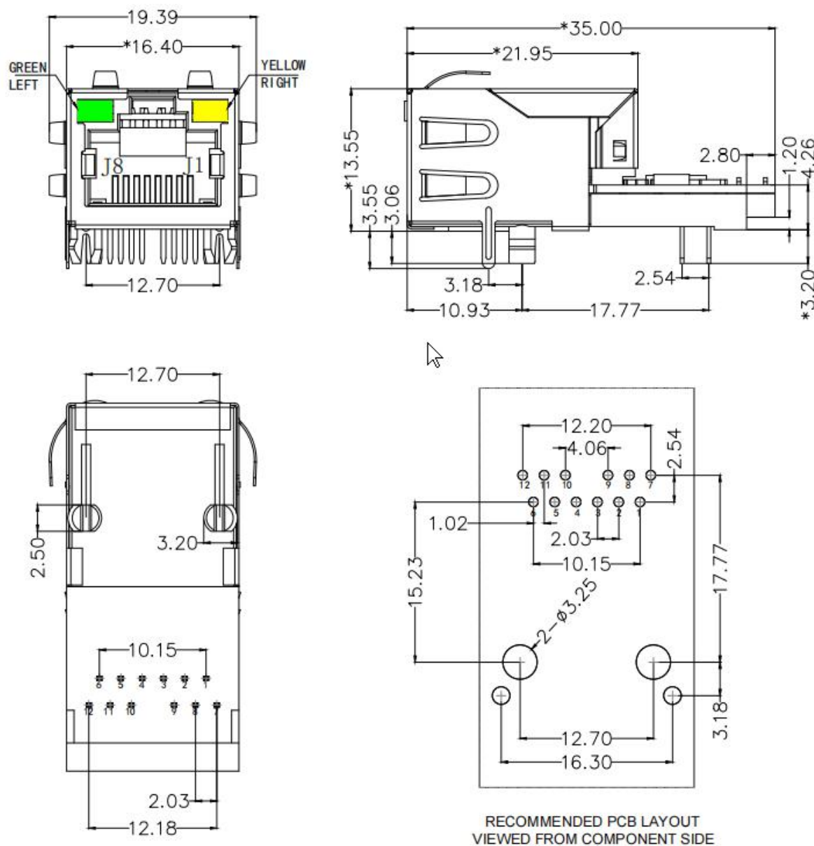
图 8 尺寸图
