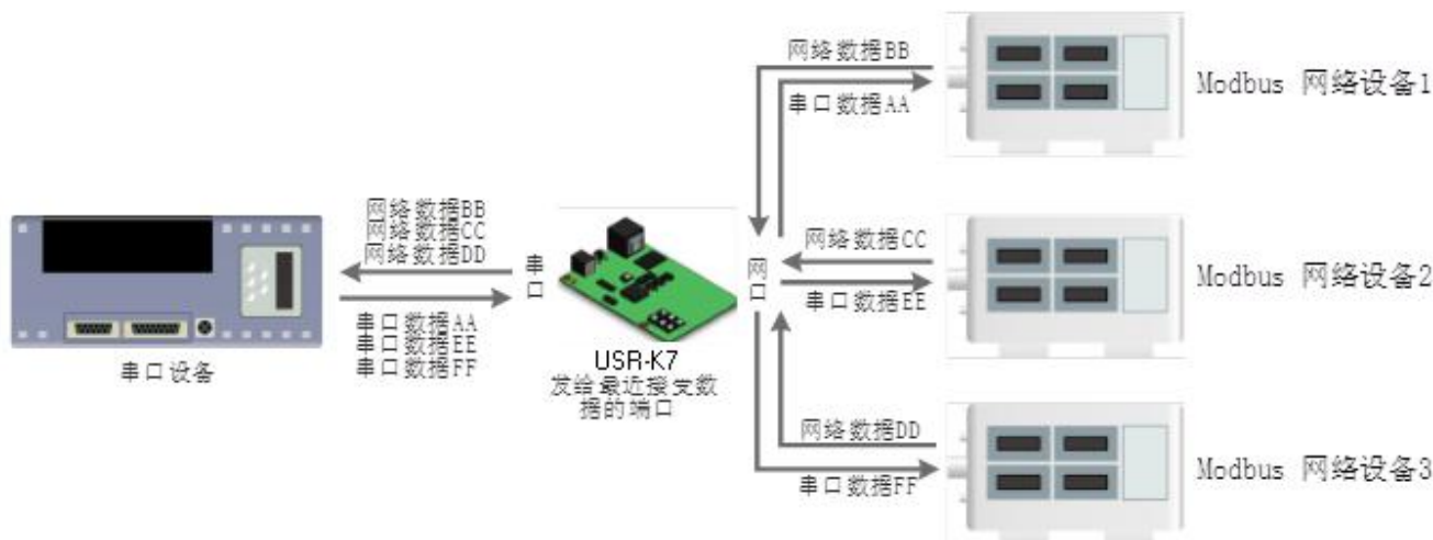
图 31 Modbus TCP 轮询
