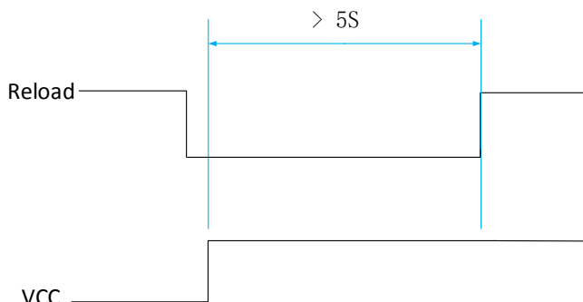
图4 恢复出厂设置时序图
