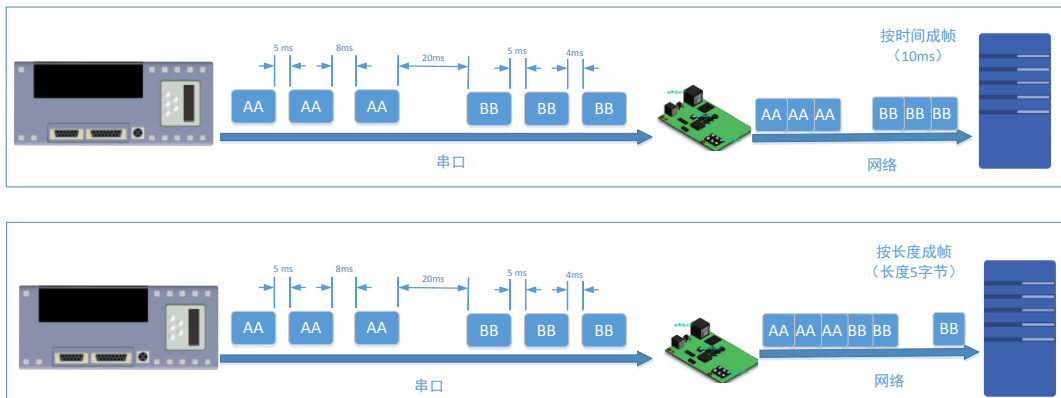
图32 串口成帧说明
