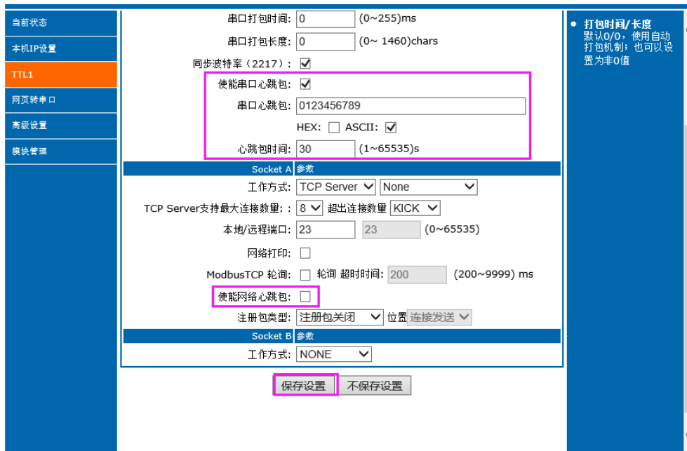
图35 心跳包功能设置
