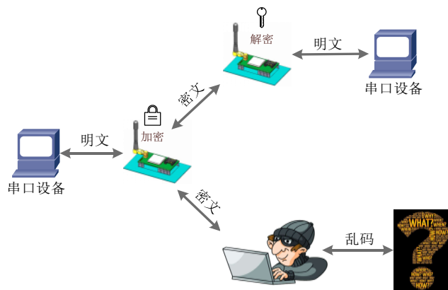
图 44 数据加密
