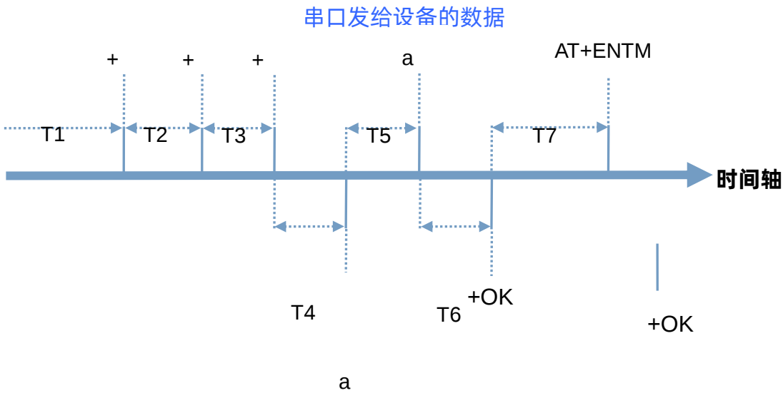
图 46 切换指令模式时序
