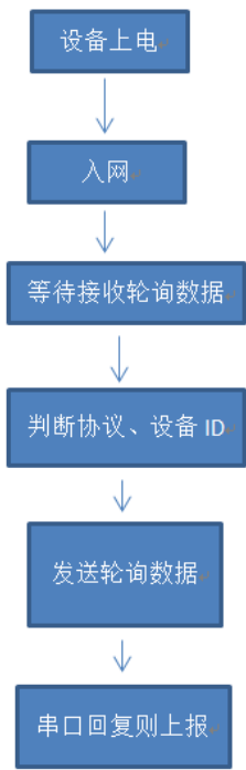
图 17 被动轮询简易流程
