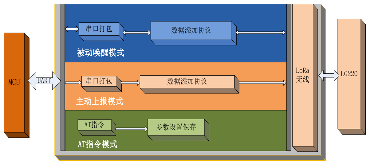
图 3 功能框图
