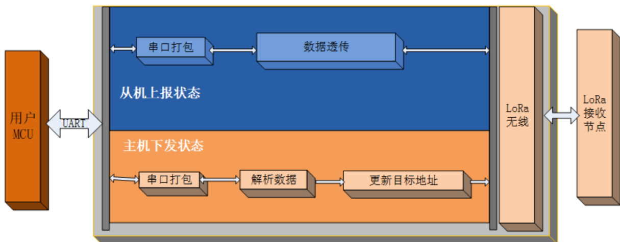
图 10 功能框图
