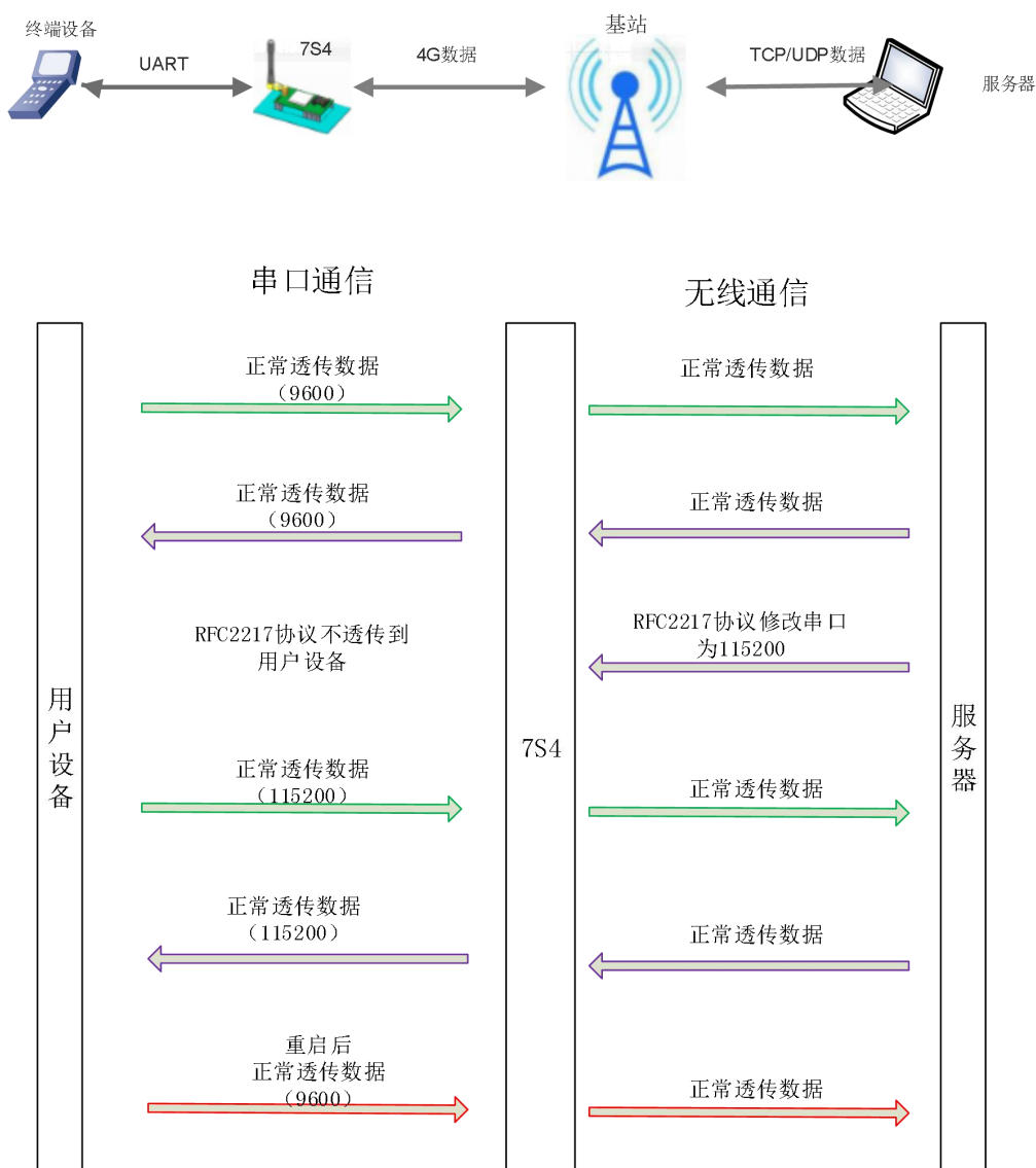
图 8 类 RFC2217
