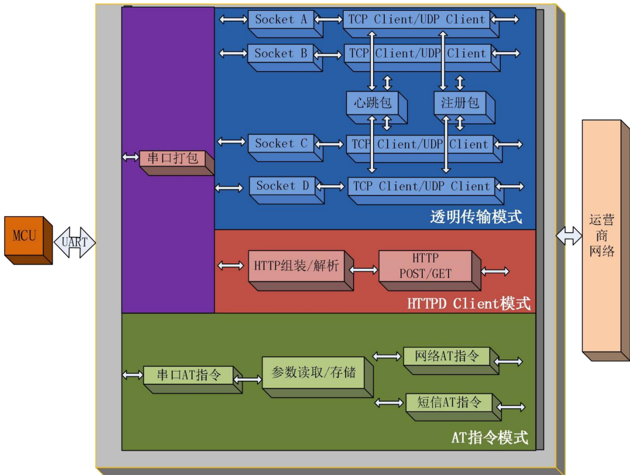
图 1 功能框图
