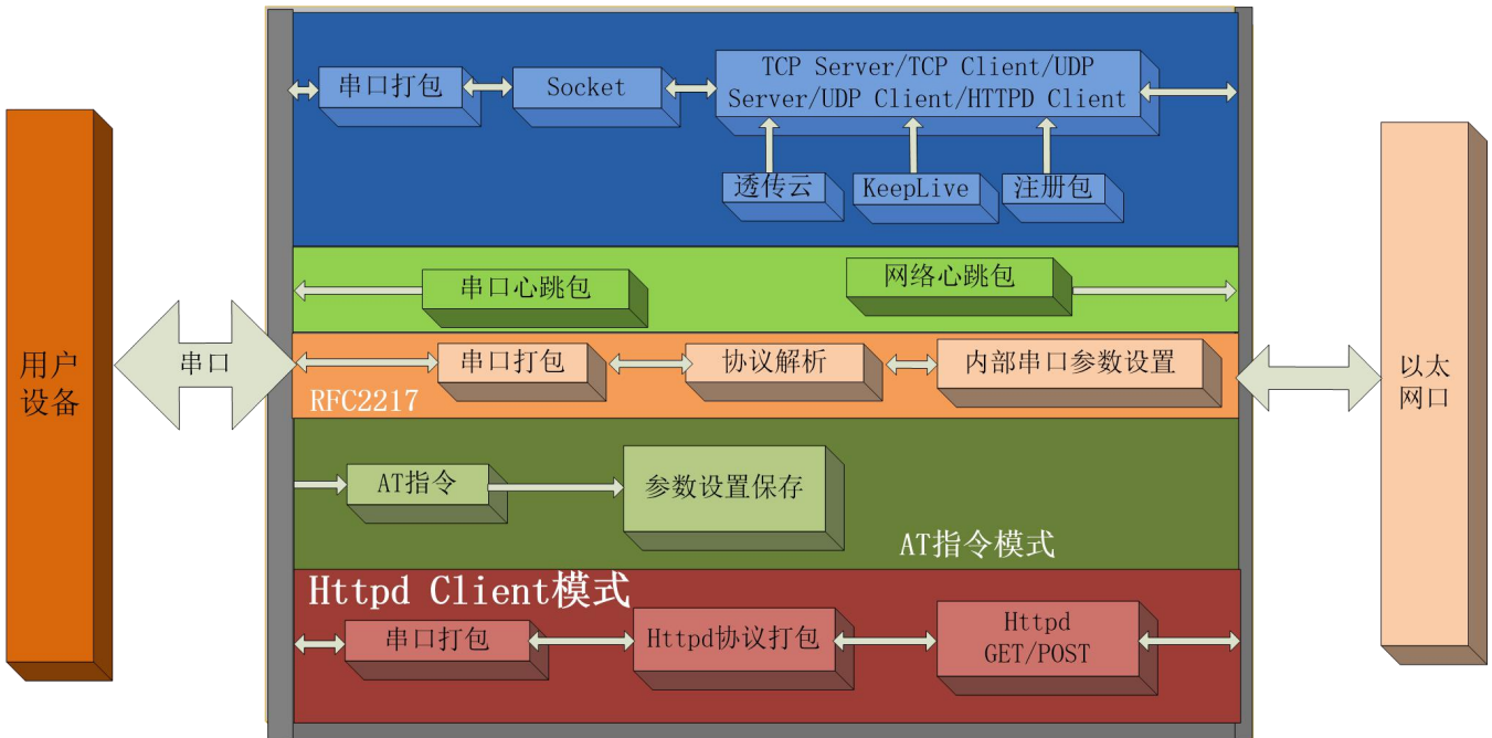
图 7. N580 功能框图
