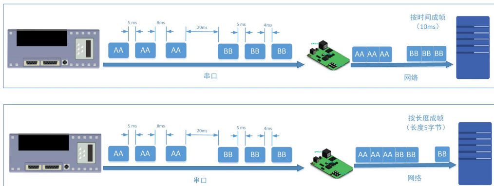
图 22. 串口成帧说明
