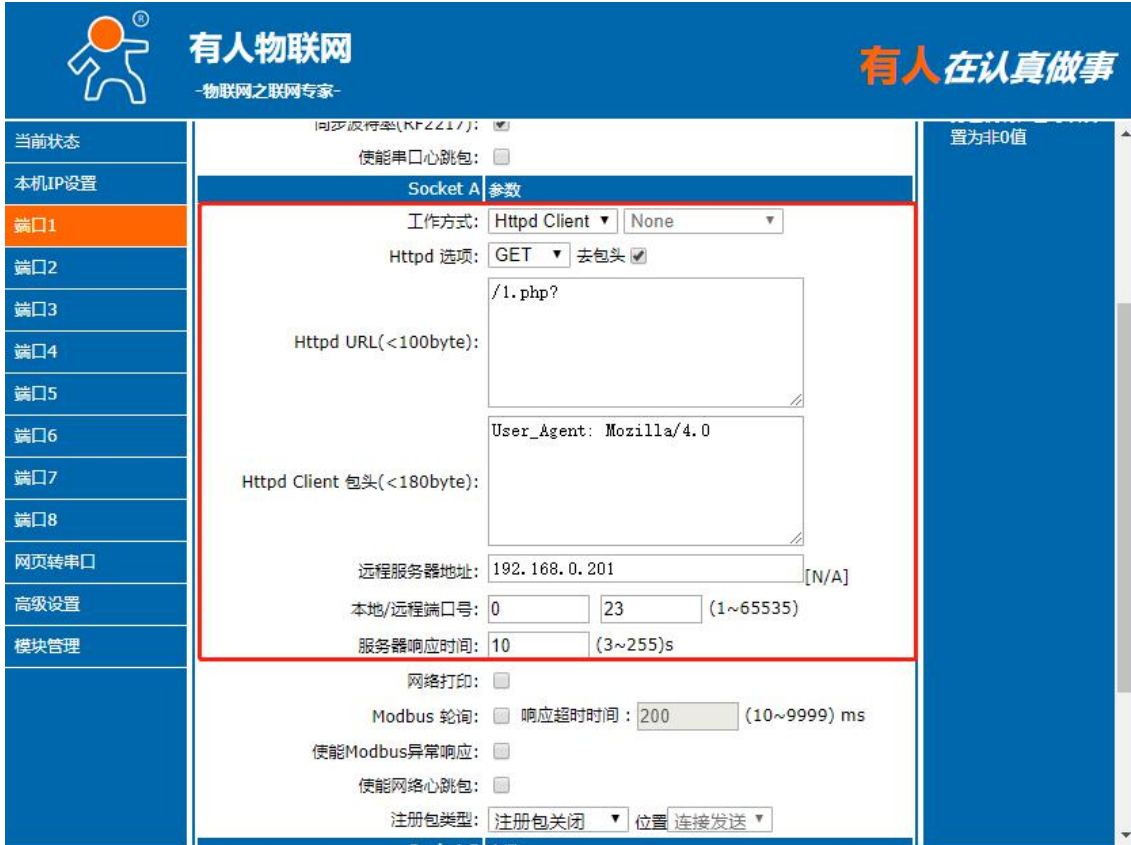
图 17. Httpd Client 模式说明
