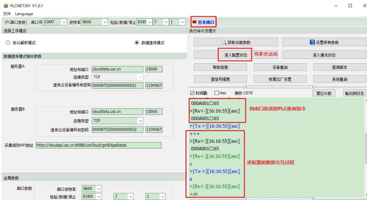
图 7 进入串口 AT 指令模式
