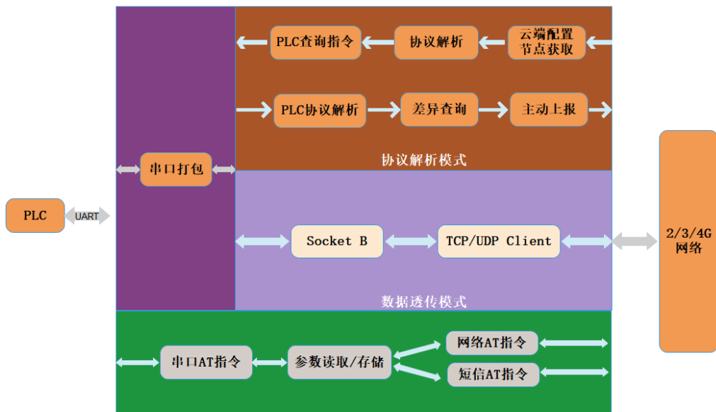
图 2 功能框图
