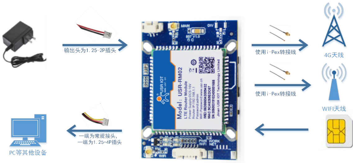
图 3 应用示意图
