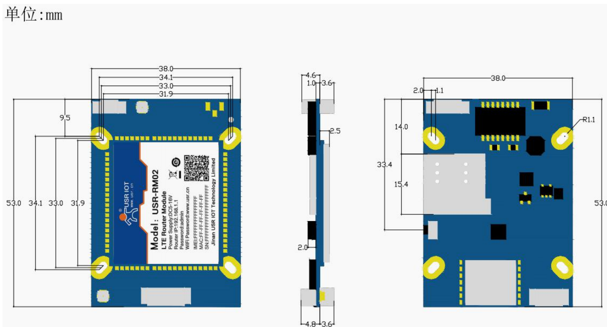
图 1 USR-RM02 尺寸图
