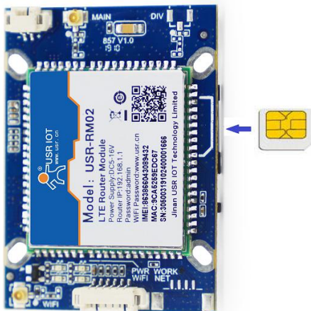
图 4 SIM 卡插入方向
