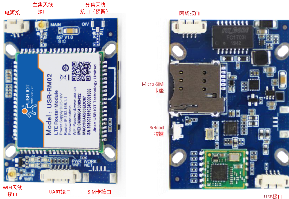
图 2 RM02 接口总览（正面/反面）
