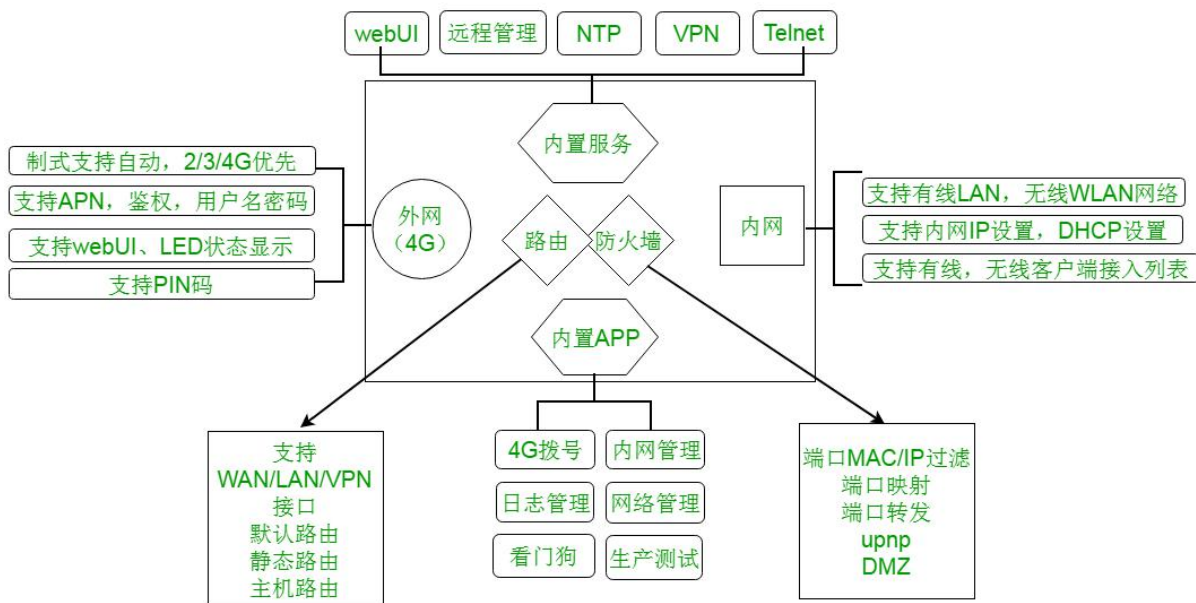
图 6 功能框图
