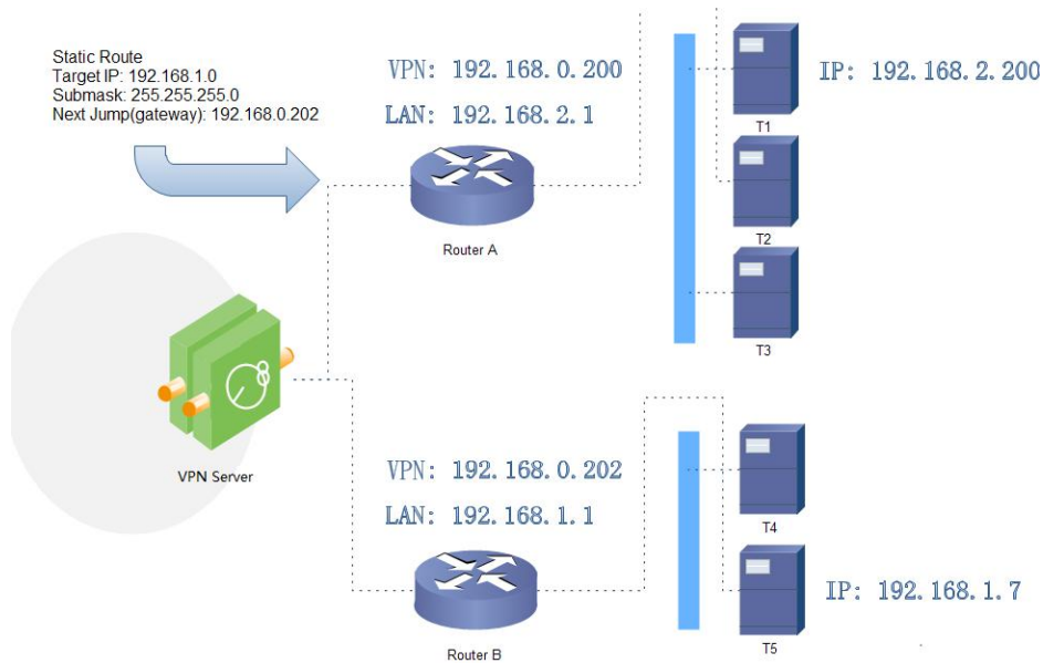
图 36 静态路由表实例图
