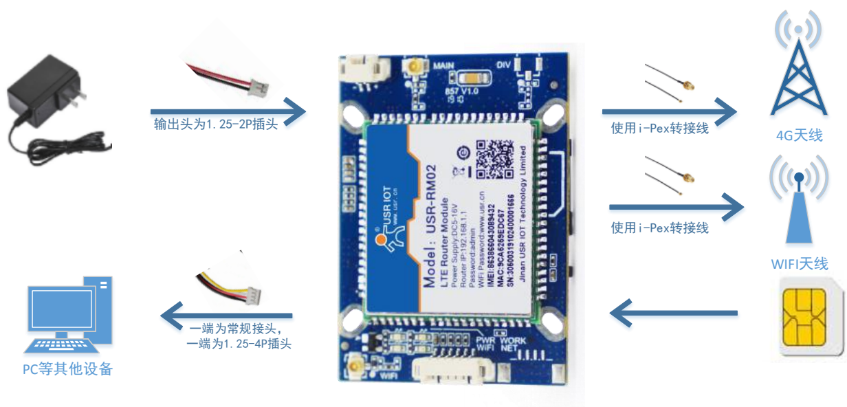
图 1 应用示意图
