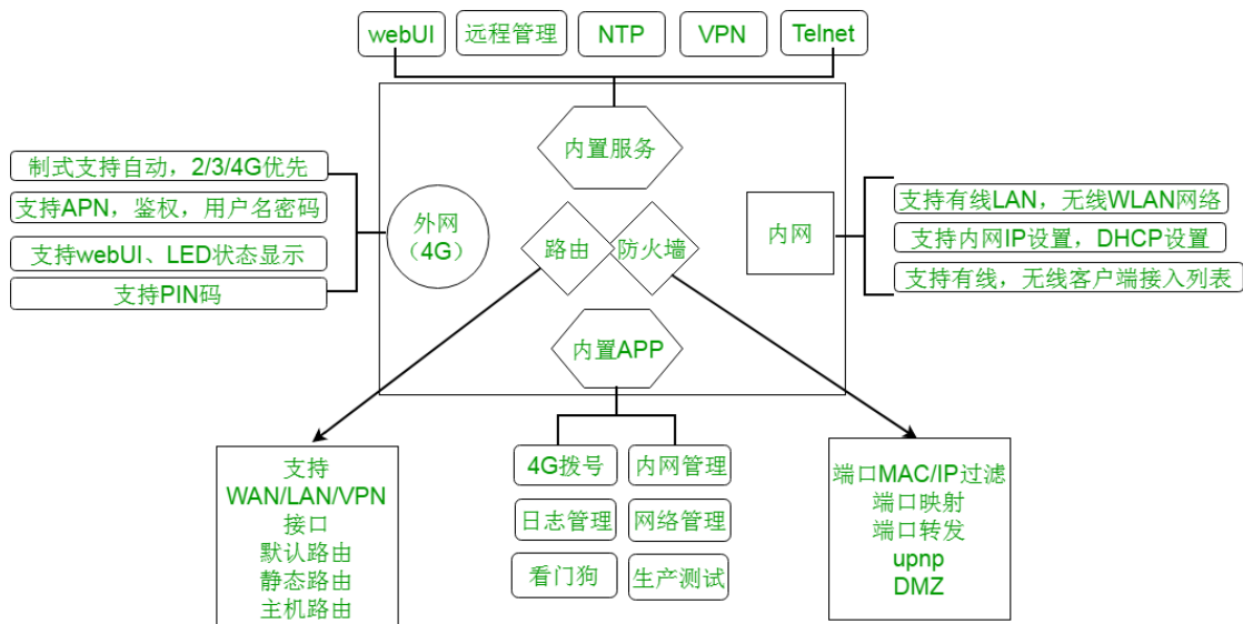
图 4 功能框图
