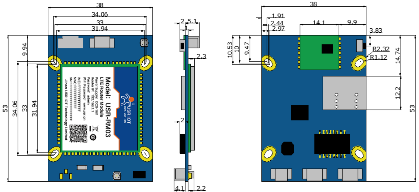
图 1 USR-RM03 尺寸图
