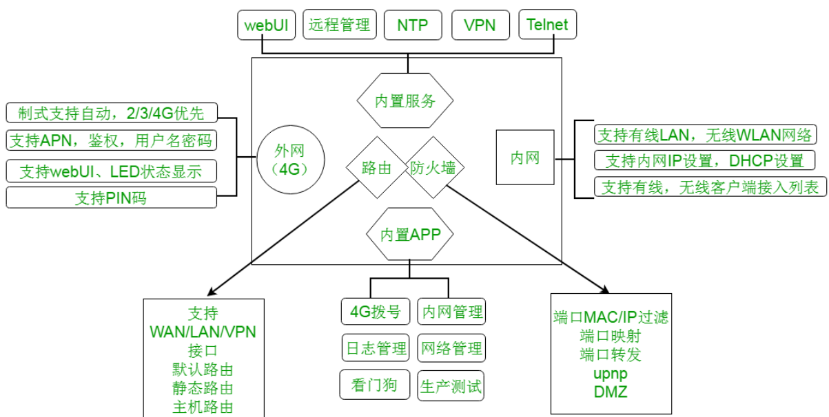
图 6 功能框图
