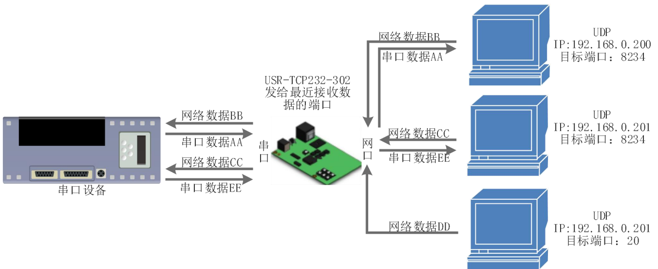
UDP Server 模式说明
