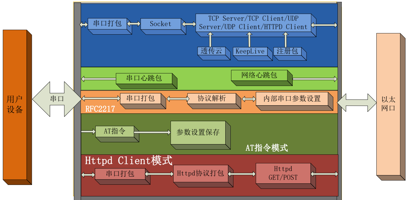
302 功能框图
