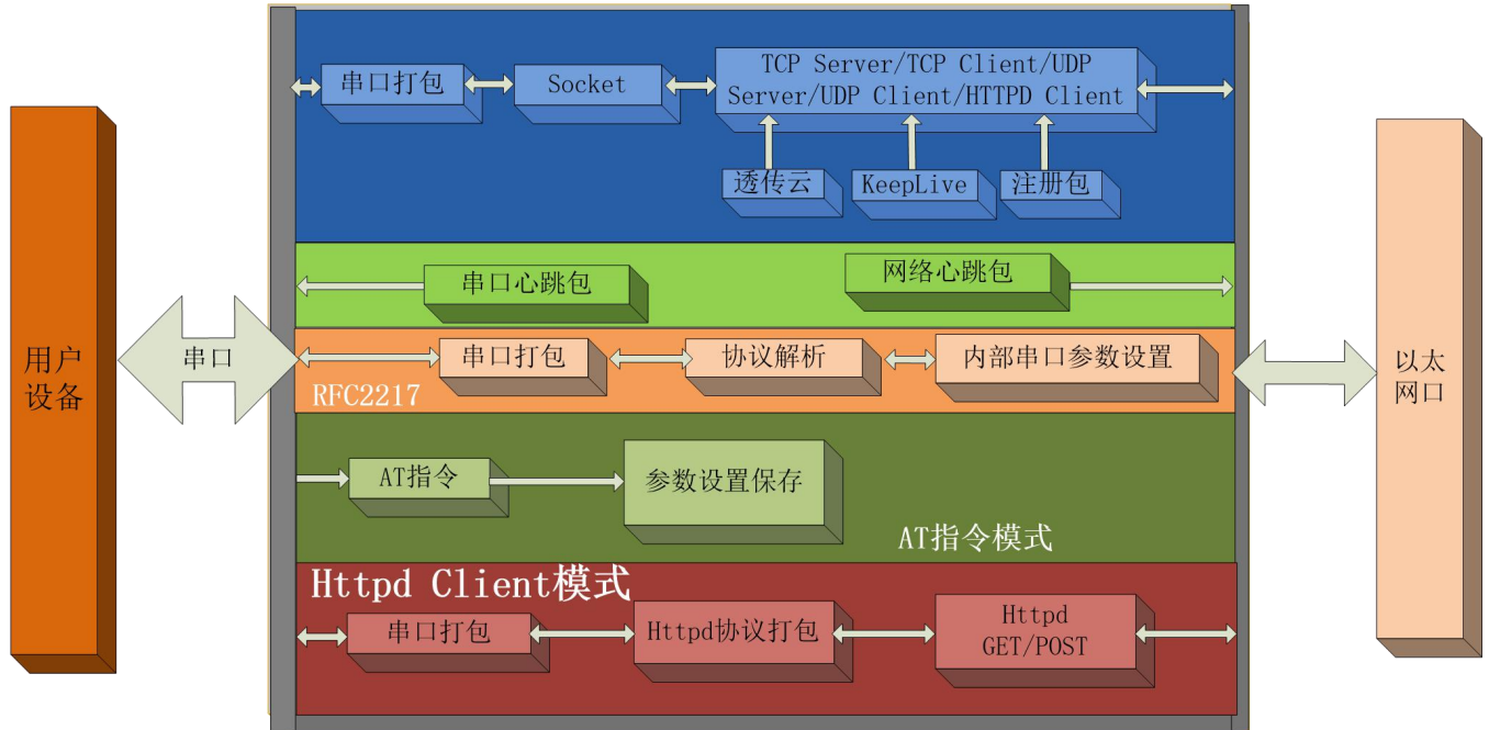
图 1. 304 功能框图
