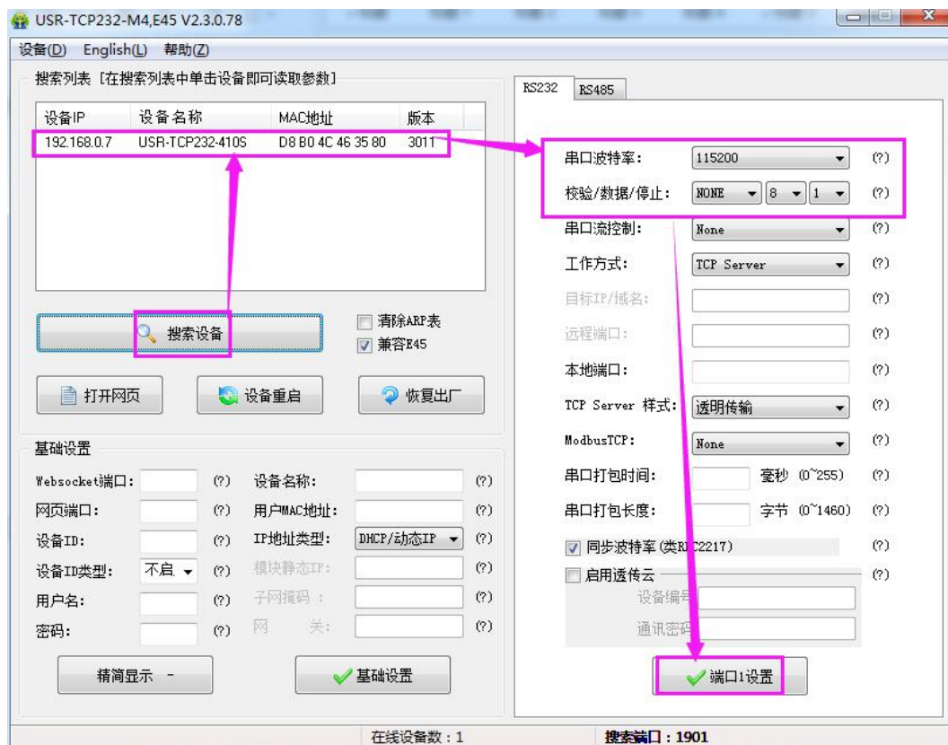
图 21 串口基本参数介绍
