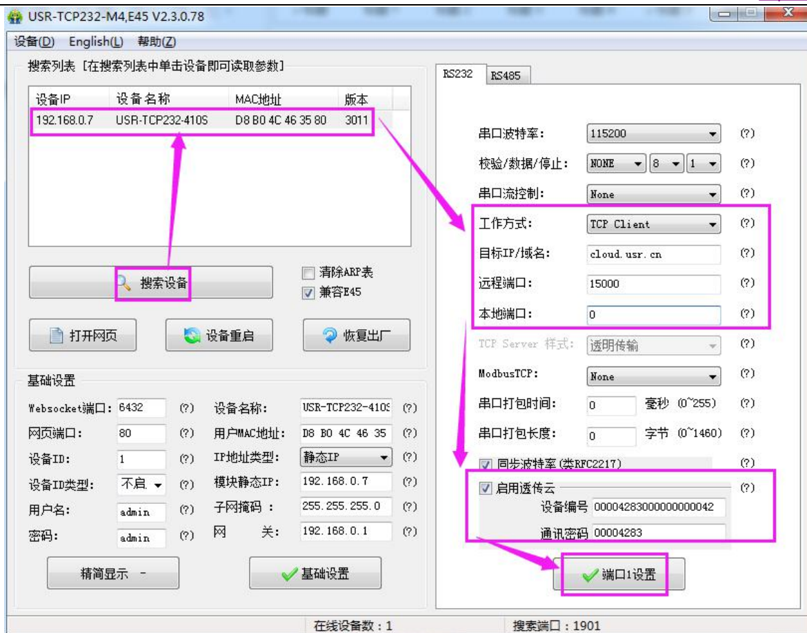
图 34 透传云设置图示
