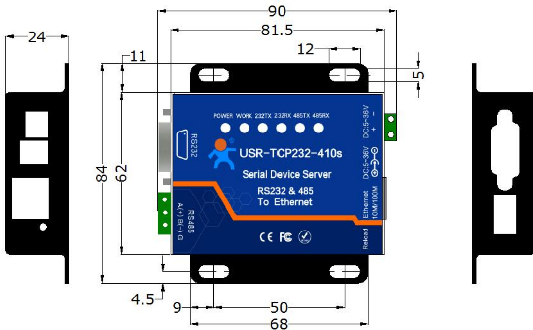
图 7 尺寸图
