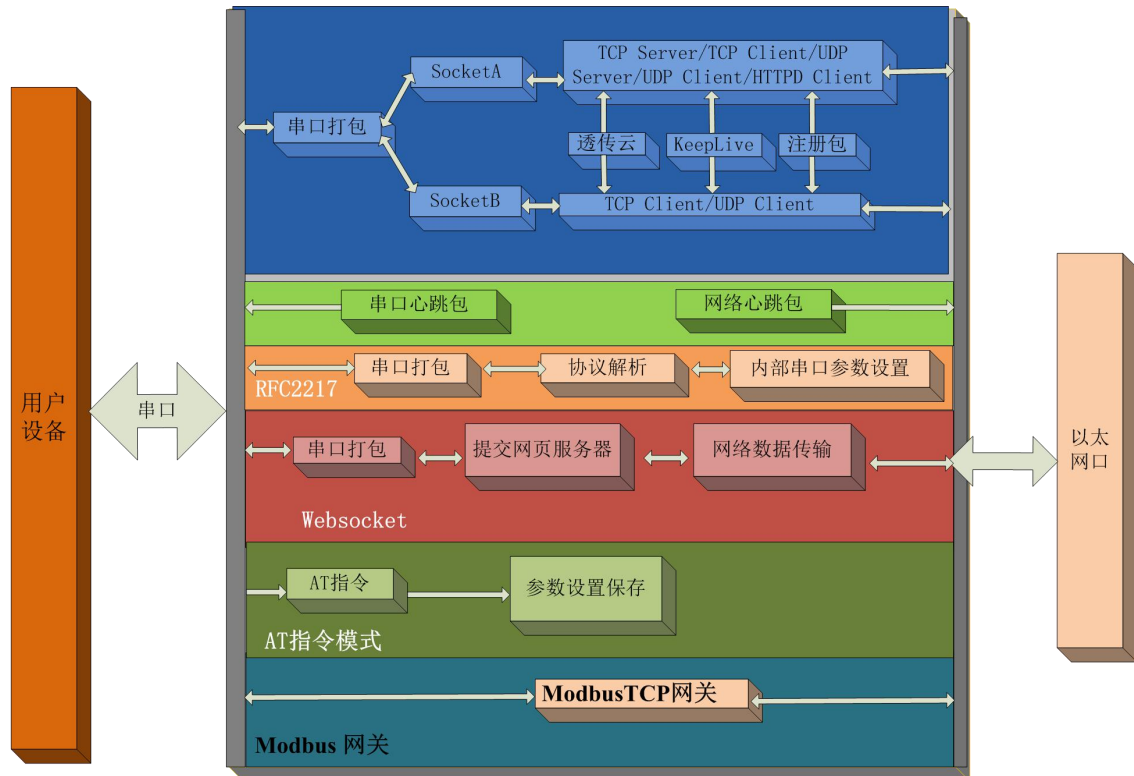
图 8 410s 功能框图
