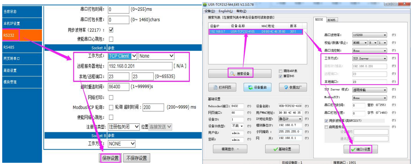
图 12 工作模式设置示例
