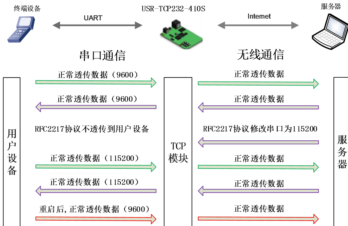
图 25 类 RFC2217 功能框图
