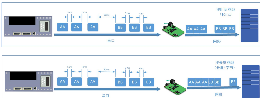
图 23 串口成帧说明
