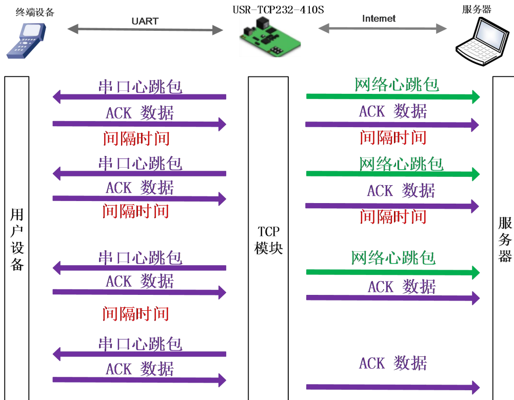
图 26 心跳包功能示意图
