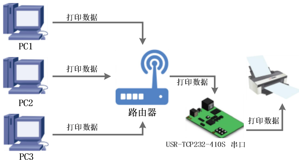
图 35 网络打印功能
