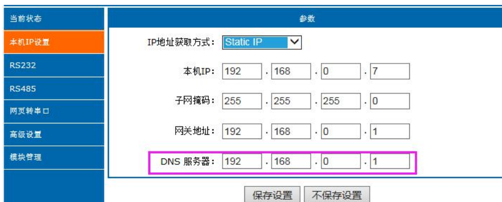
图 10 DNS 服务器
