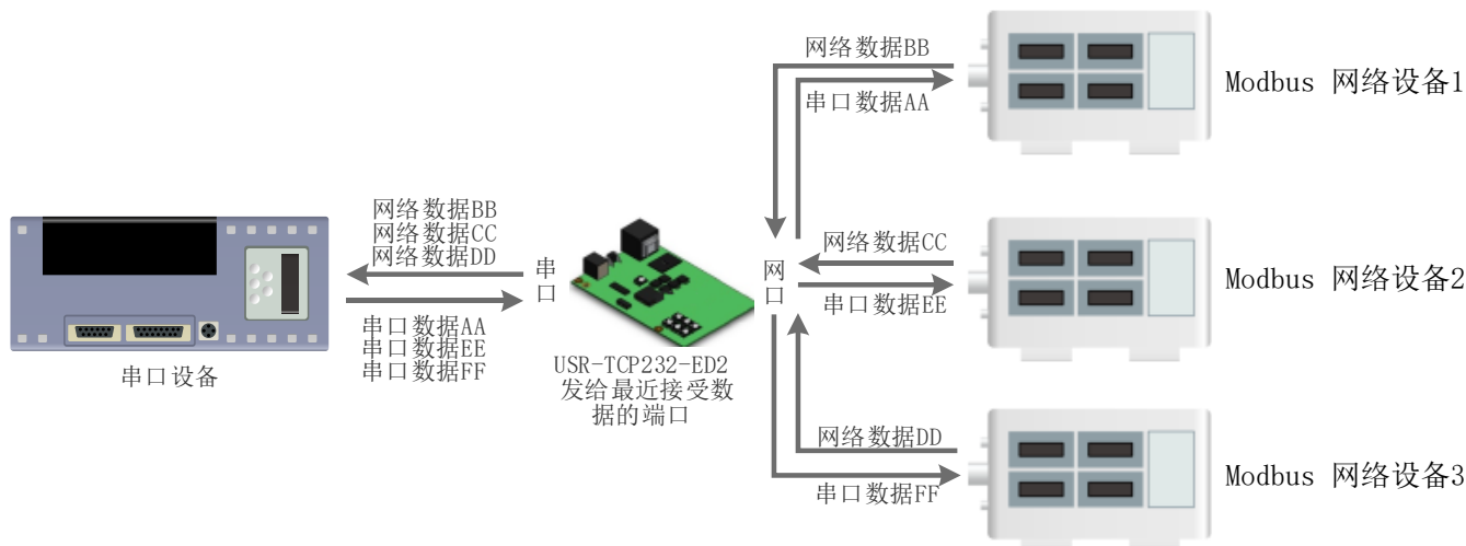
图43 Modbus TCP
