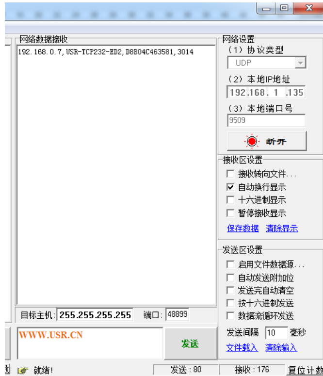
图65 网络 AT 指令图示
