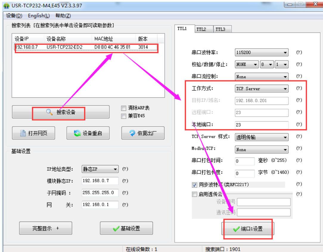
图13 TCP Server 软件设置图
