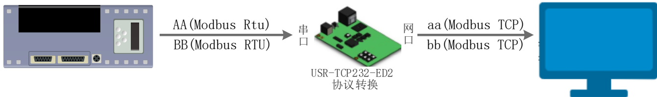
图36 Modbus TCP
