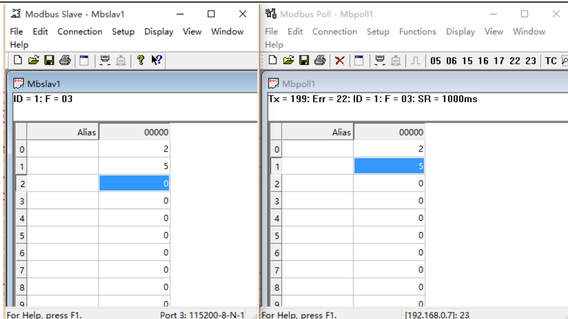
图39 Modbusrtu 转 Modbus tcp 转换结果
