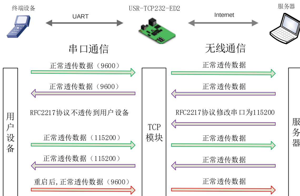
图33 RFC2217 功能框图
