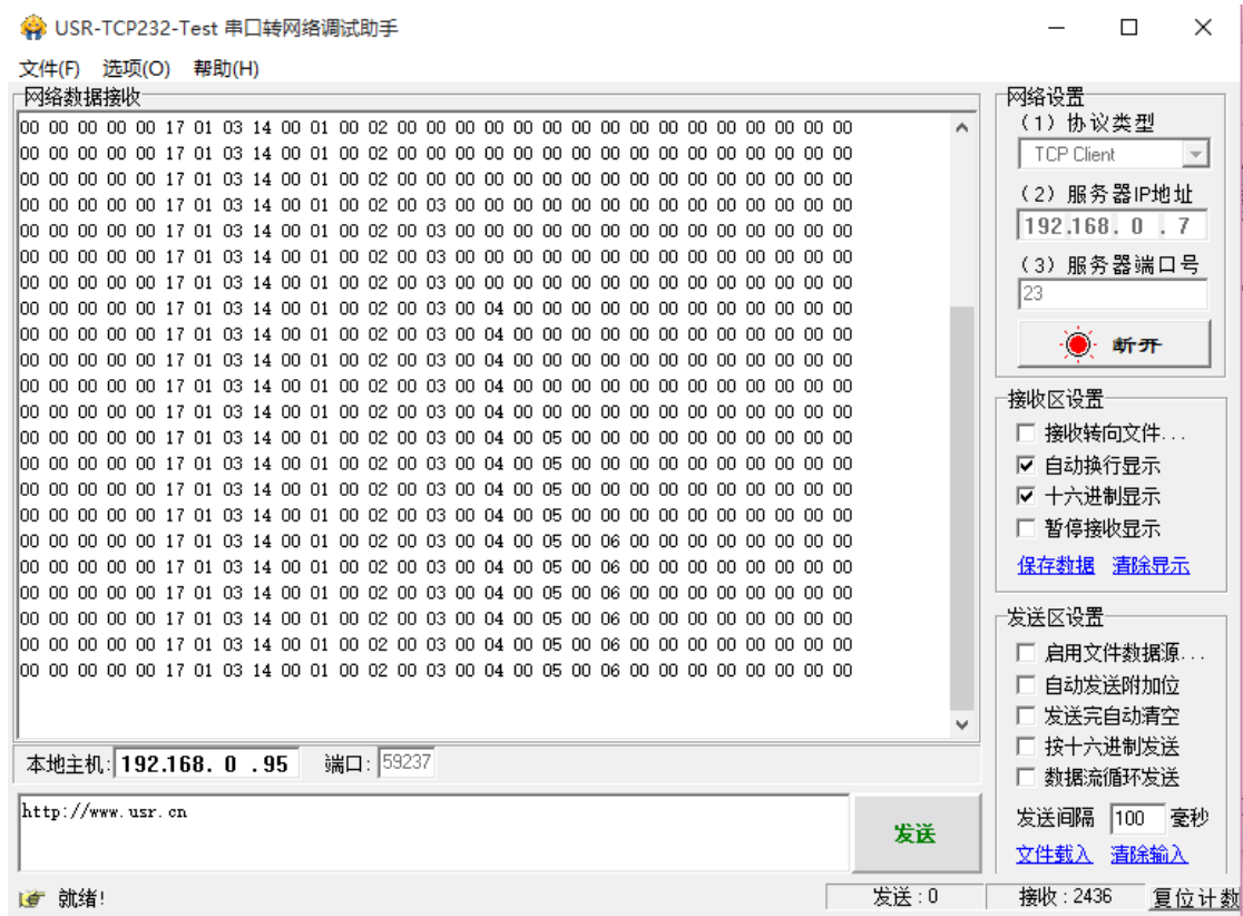
图42 Modbusrtu 主动查询设置截图
