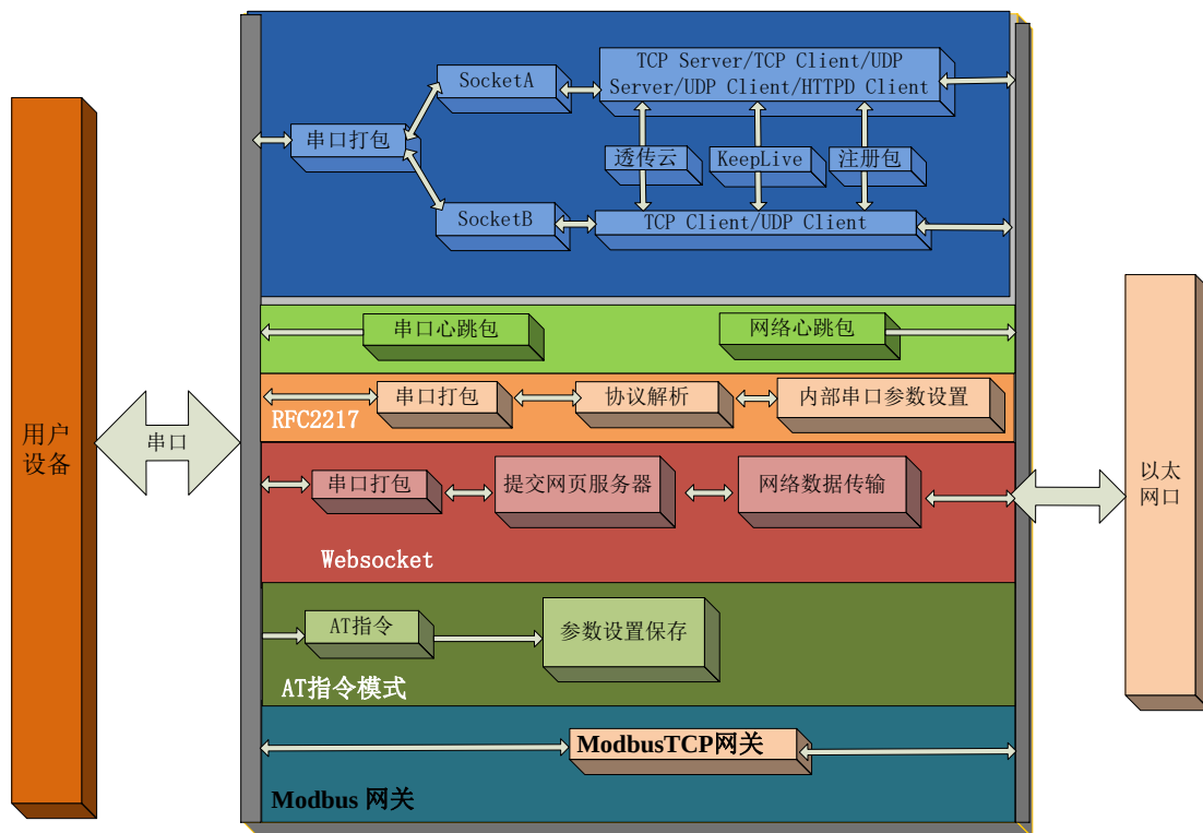
图1 ED2 功能框图
