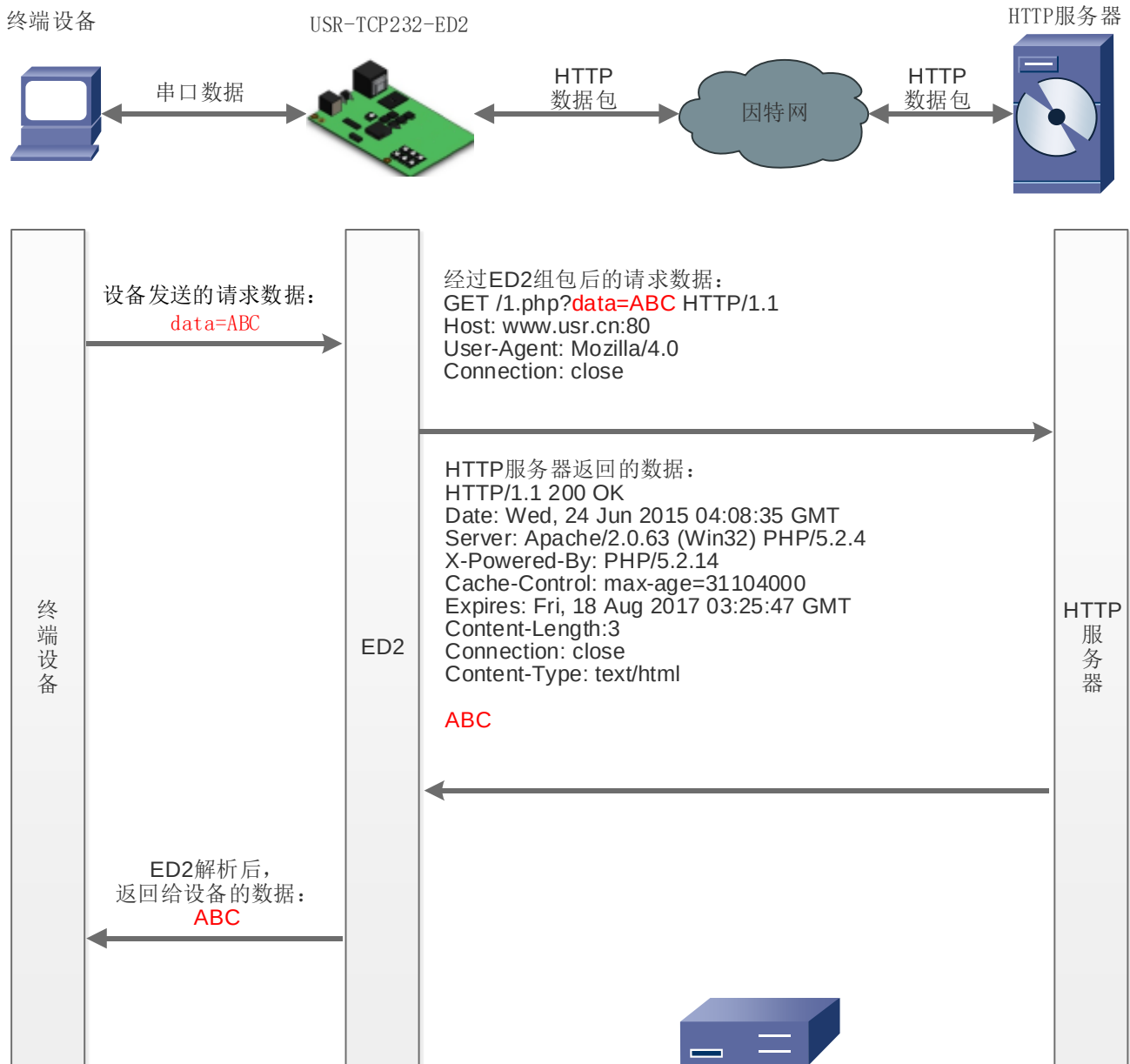
图26 Httpd Client 模式说明
