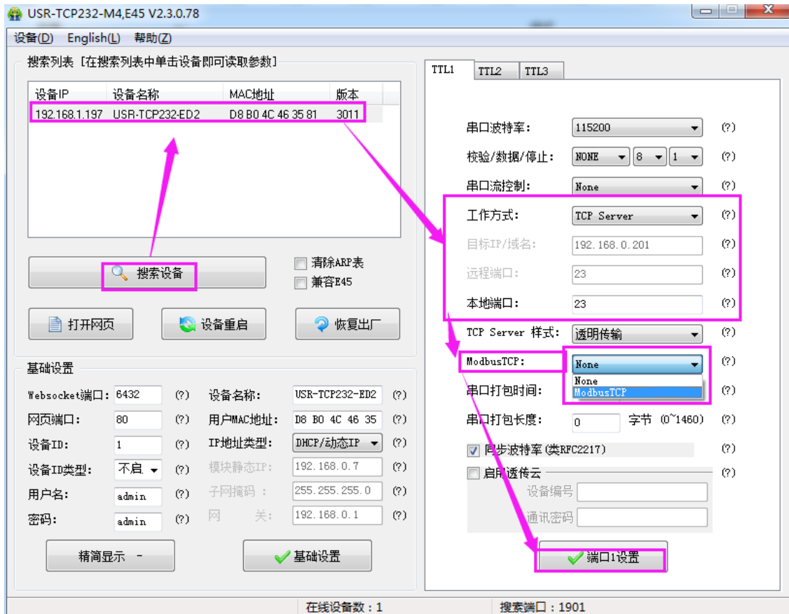
图37 Modbusrtu 转 Modbus tcp
