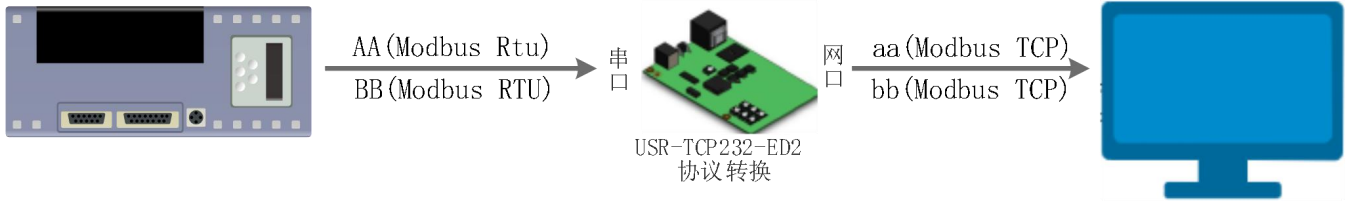
图 29 Modbus TCP
