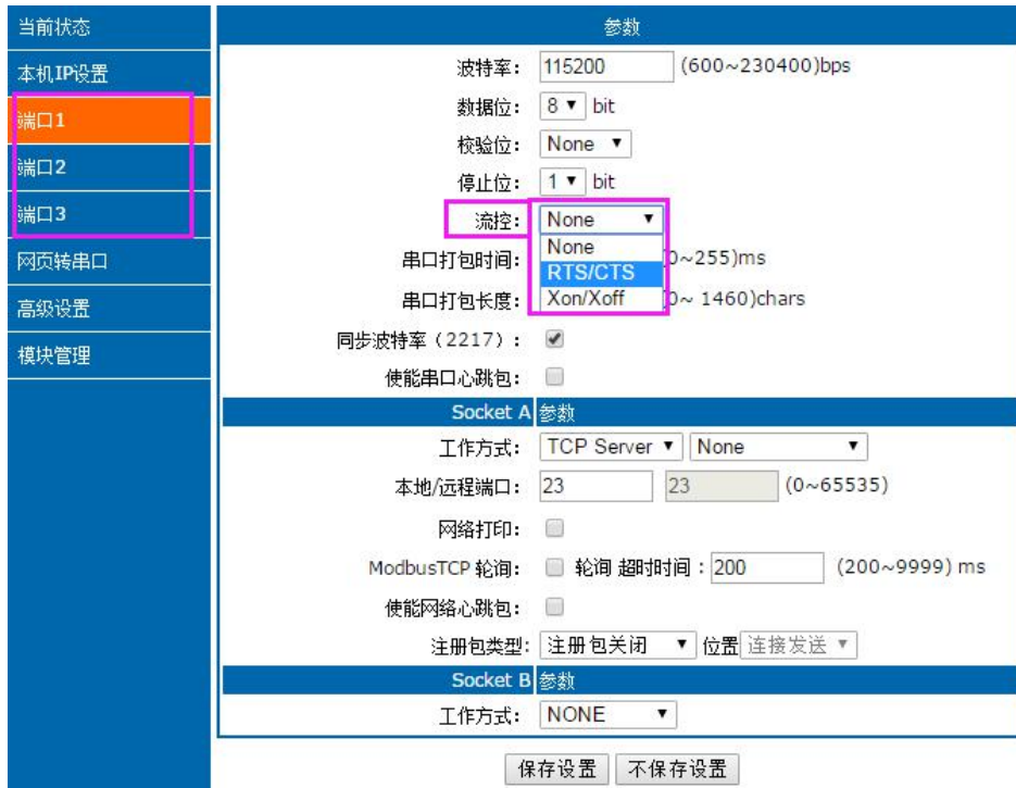
图 23 串口流控模式
