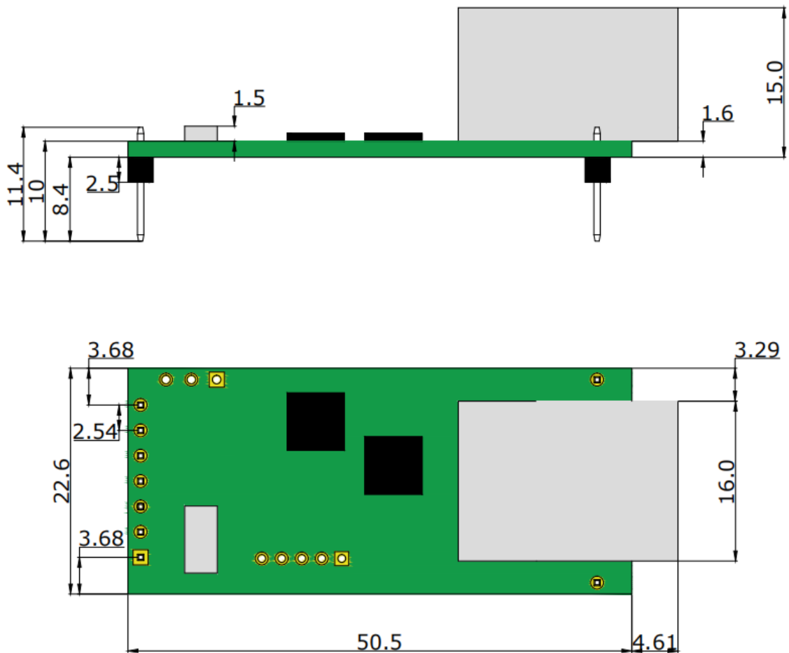
图 2 USR-TCP232-T2 尺寸图
