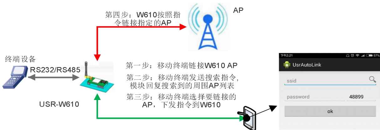
图 31 usr-link 框图
