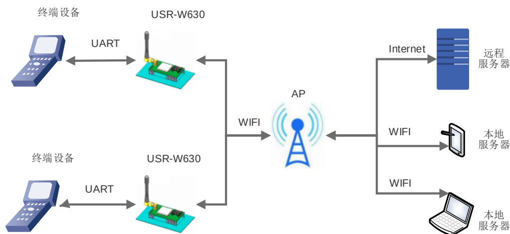
图 3 串口服务器作为 AP+STA 的应用场景
