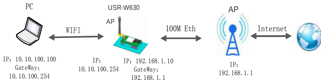
图 9 有线加无线的应用场景 3
