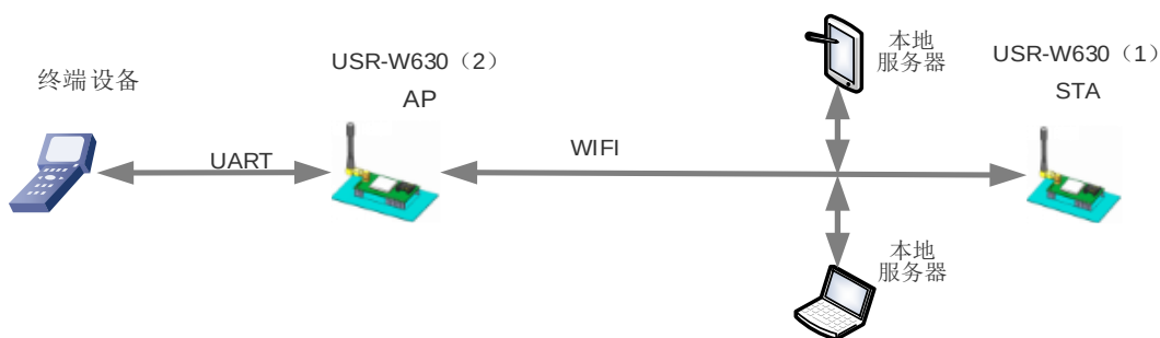
图 4 AP 与 STA 应用场景
