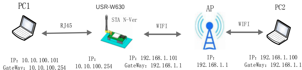
图 10 有线加无线组网应用（路由）
