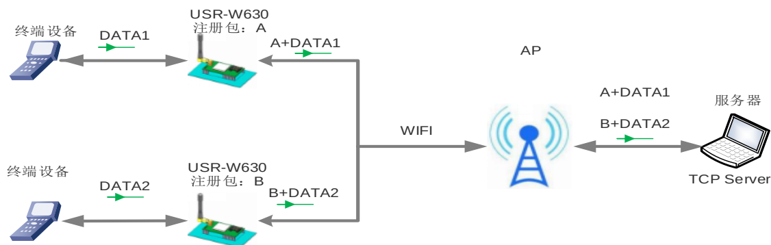
图 21 首次连接发送注册包框图
