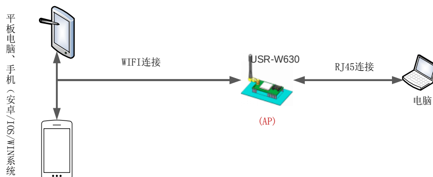
图 7 有线加无线的应用场景 1
