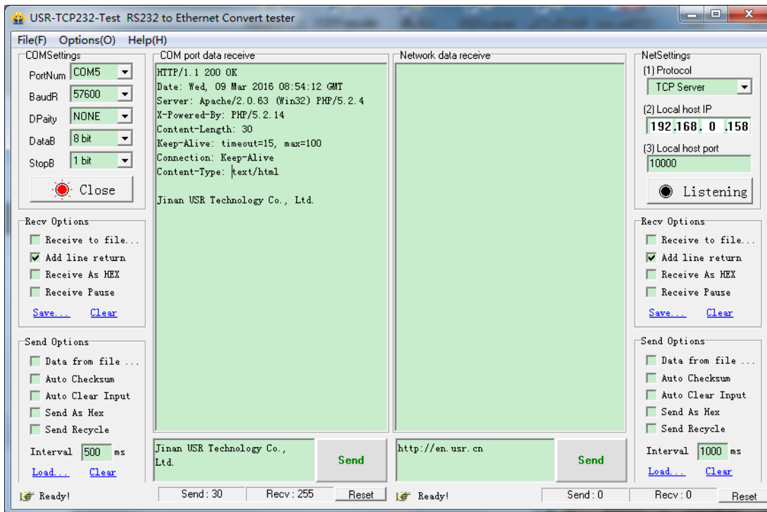
图 45 HTTPD Client 模式测试示例
