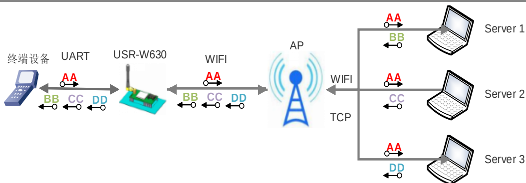
图 17 多 TCP 链接数据传输图示
