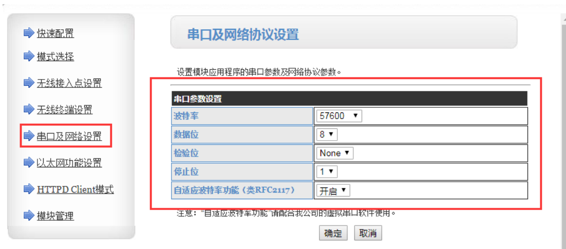
图 18 网页设置串口参数
