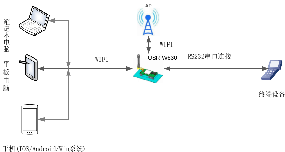
图 6 无线桥接应用场景
