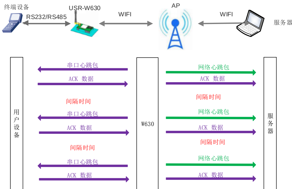
图 27 自定义心跳包功能框图
