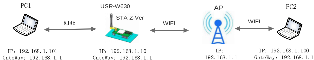
图 11 有线加无线组网应用（桥接）
