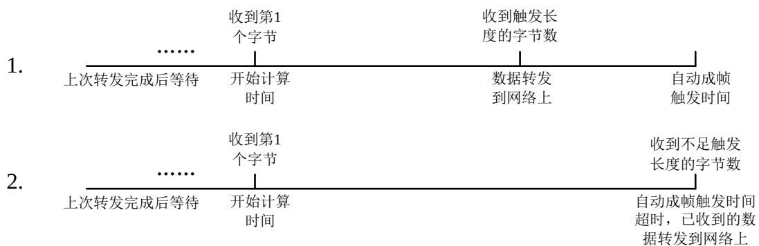
图 20 自动成帧功能示意图
