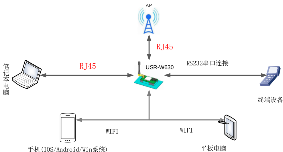
图 5 网线桥接应用场景
