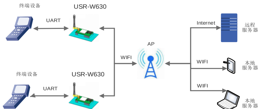
图 2 串口服务器作为 STA 的应用场景
