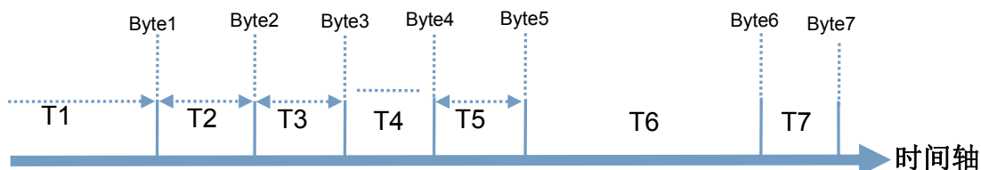
图 14 切换指令模式时序
