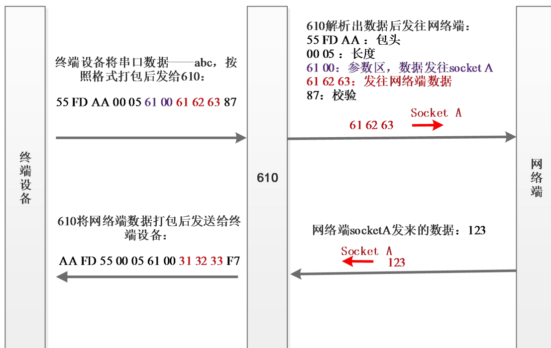
图 20 套接字分发框图
