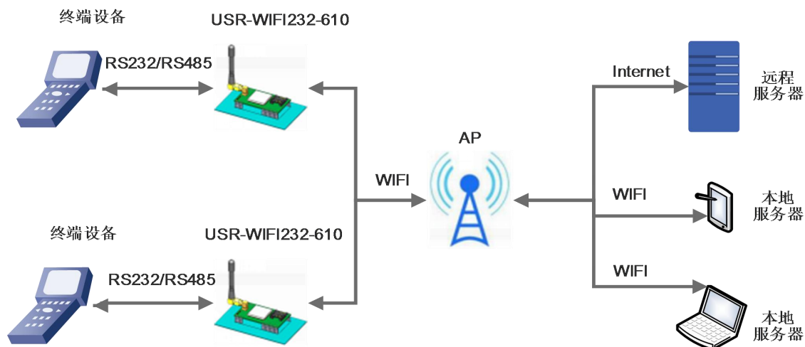
图 4 无线组网应用（STA）
