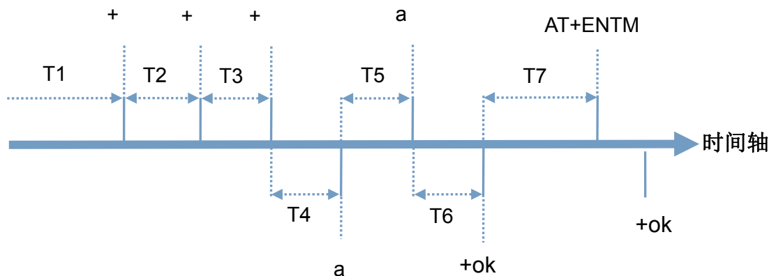
图 32 进入串口 AT 命令模式时序
