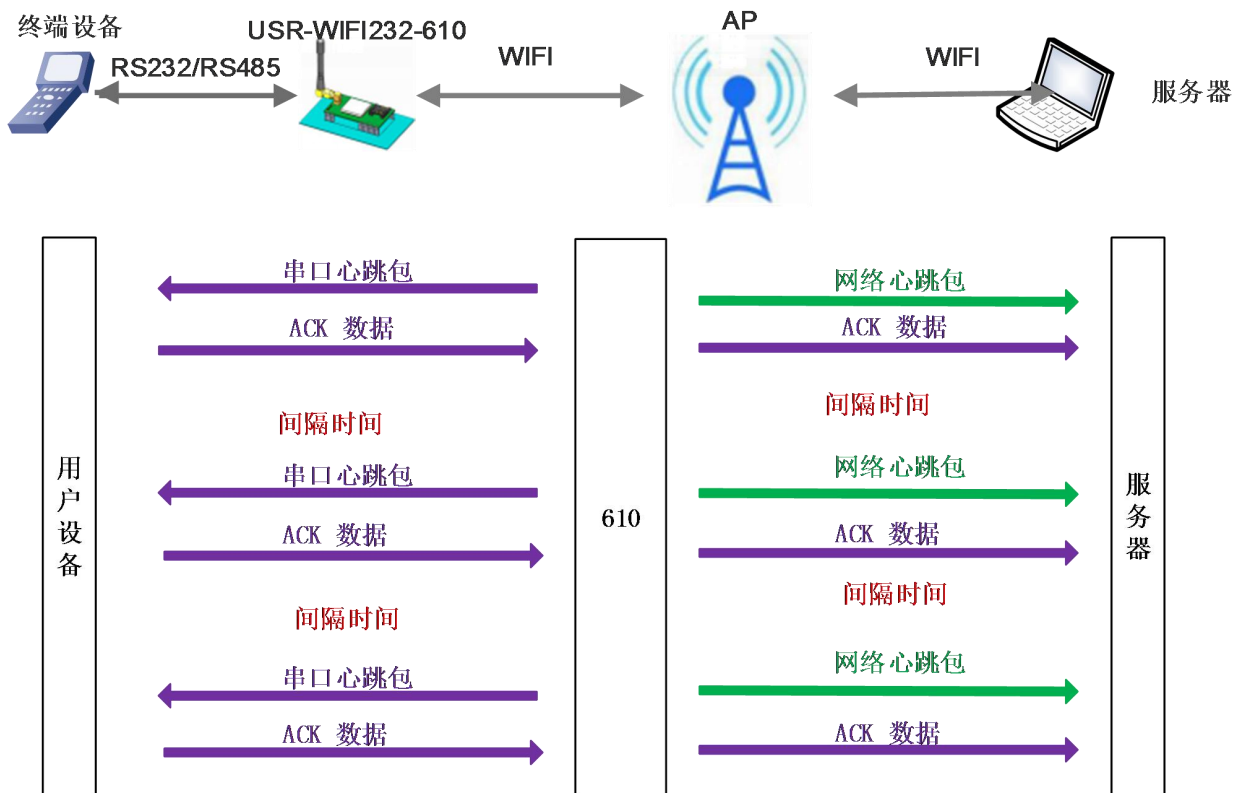
图 19 自定义心跳包功能框图
