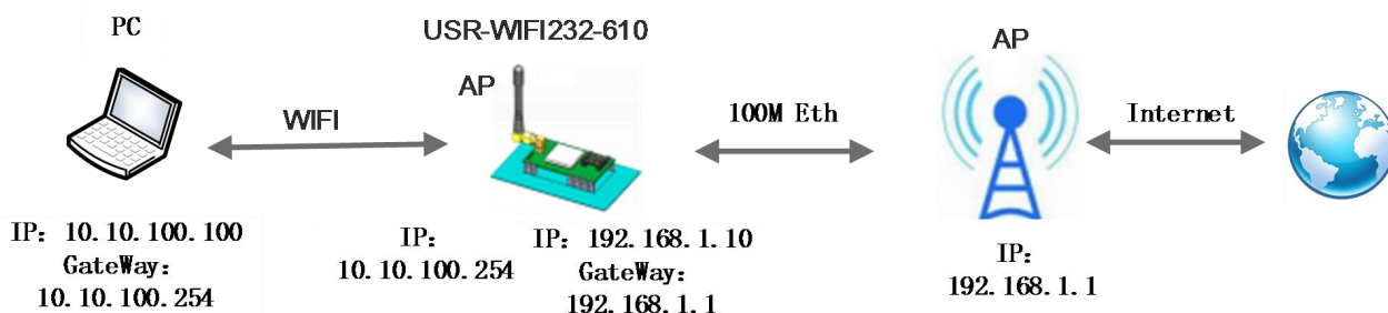
图 9 有线加无线的组网应用（AP WAN）
