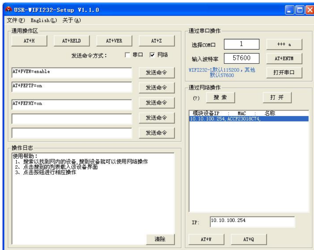
图 37 设置软件整体应用图
