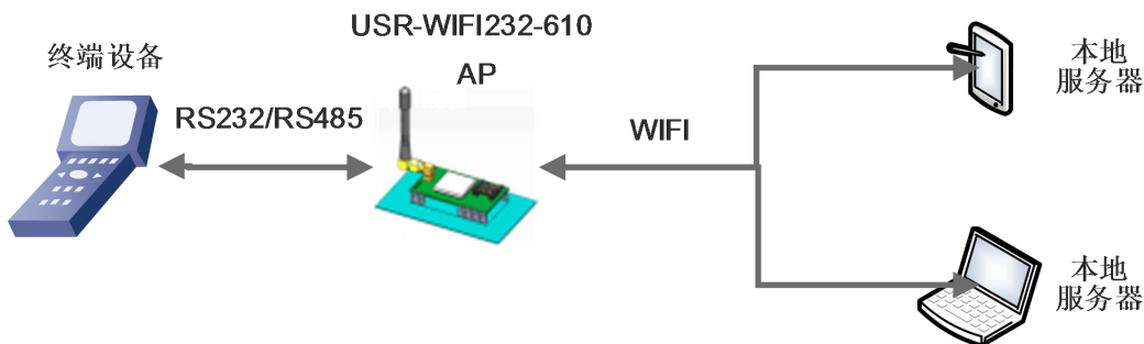
图 3 无线组网应用（AP）
