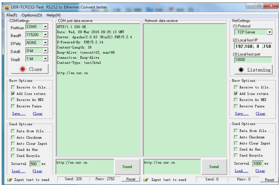
图 28 HTTPD Client 模式设置页面及测试示例
