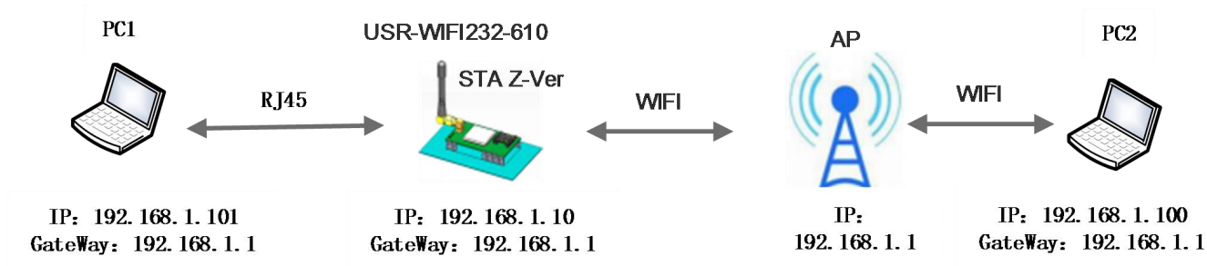
图 11 有线加无线组网应用（桥接）
