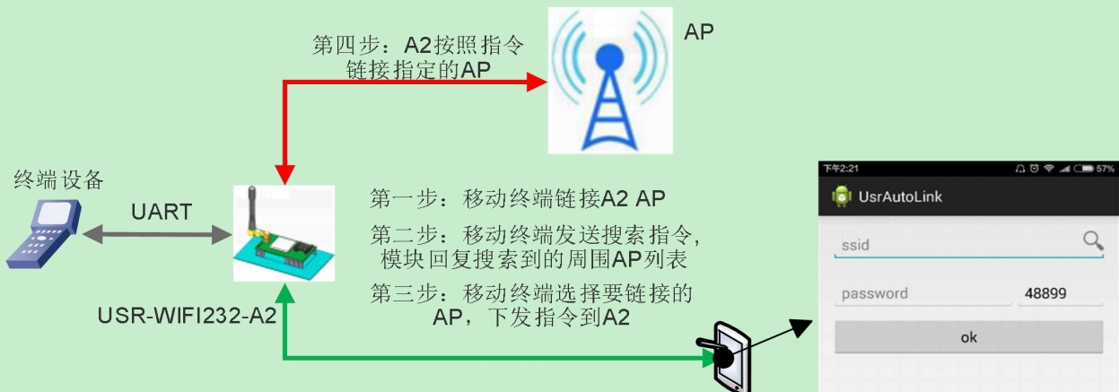
图 32 usr-link 框图
