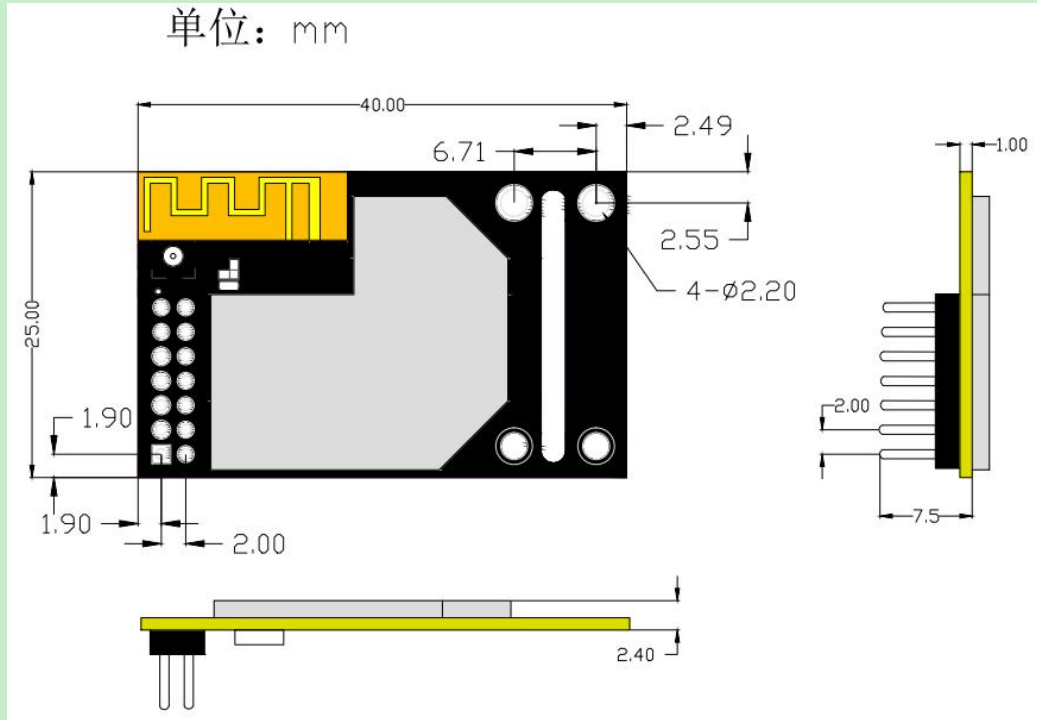
图 7 USR-WIFI232-A2 尺寸图
