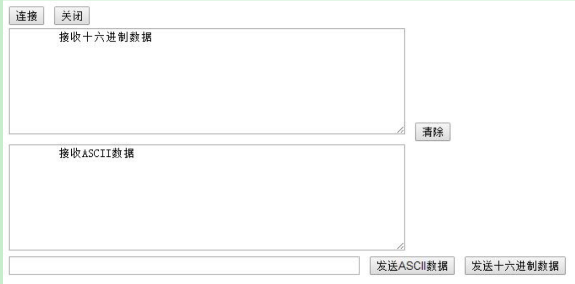
图 31 WebSocket 页面
