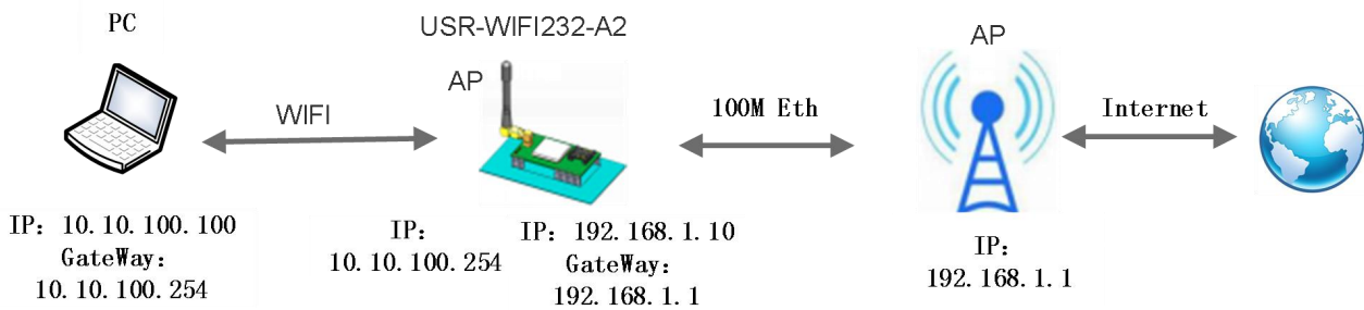
图 9 USR-WIFI232-A2 以太网接口功能（AP WAN）
