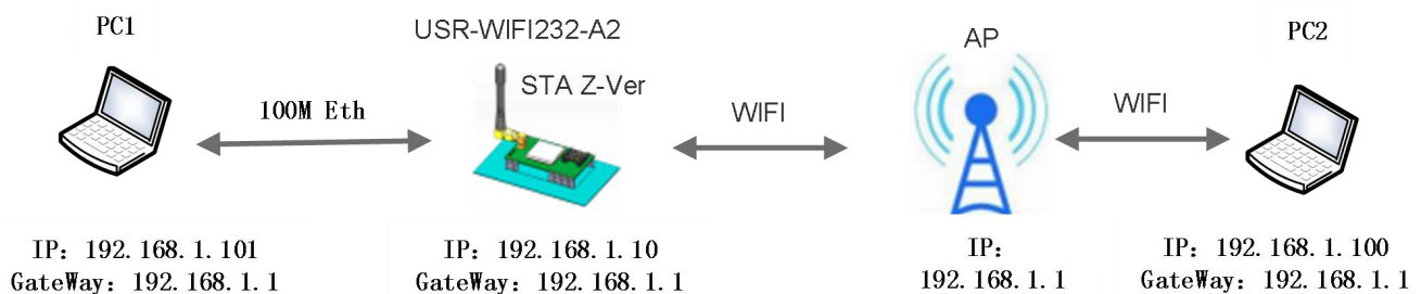
图 11 USR-WIFI232-A2 以太网接口功能（STA Z-Ver）
