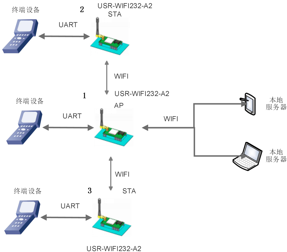
图 6 USR-WIFI232-A2 自组网 2
