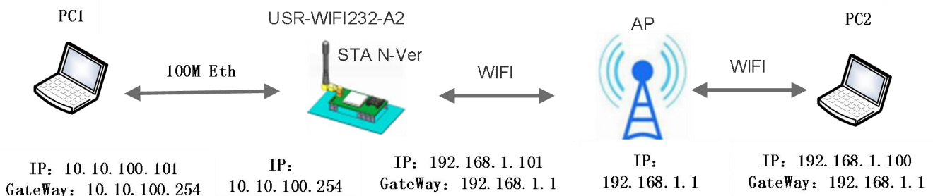
图 10 USR-WIFI232-A2 以太网接口功能（STA N-Ver）
