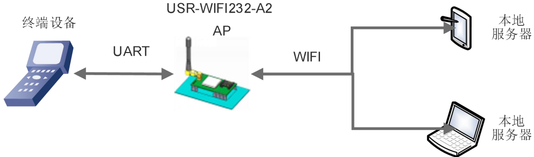
图 5 USR-WIFI232-A2 自组网 1
