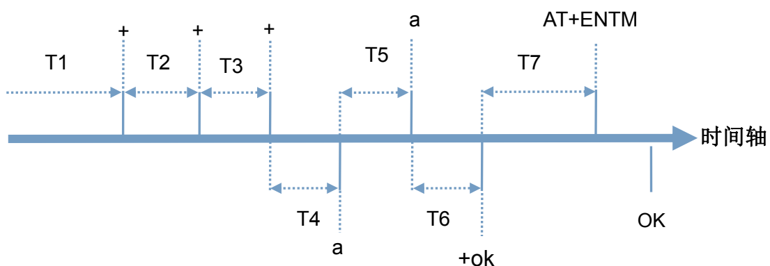
图 24. +++a 时序图
