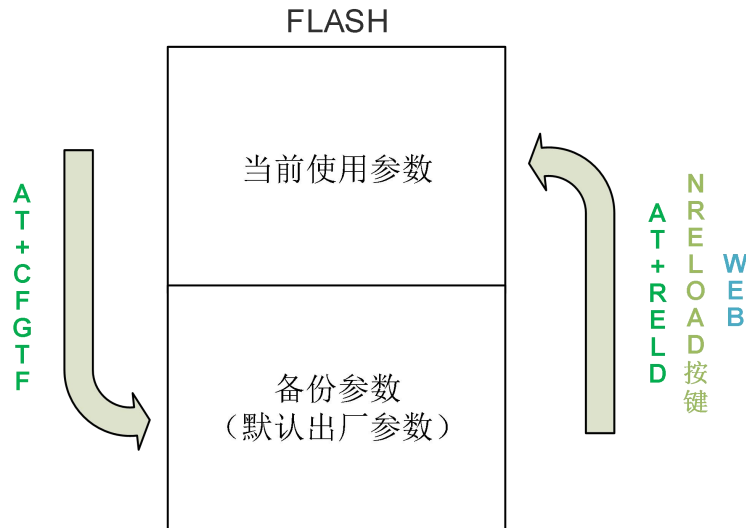
图 23 模块参数
