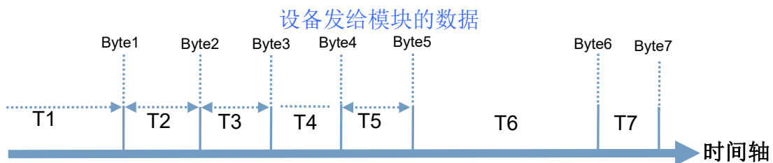
图 13 成帧机制
