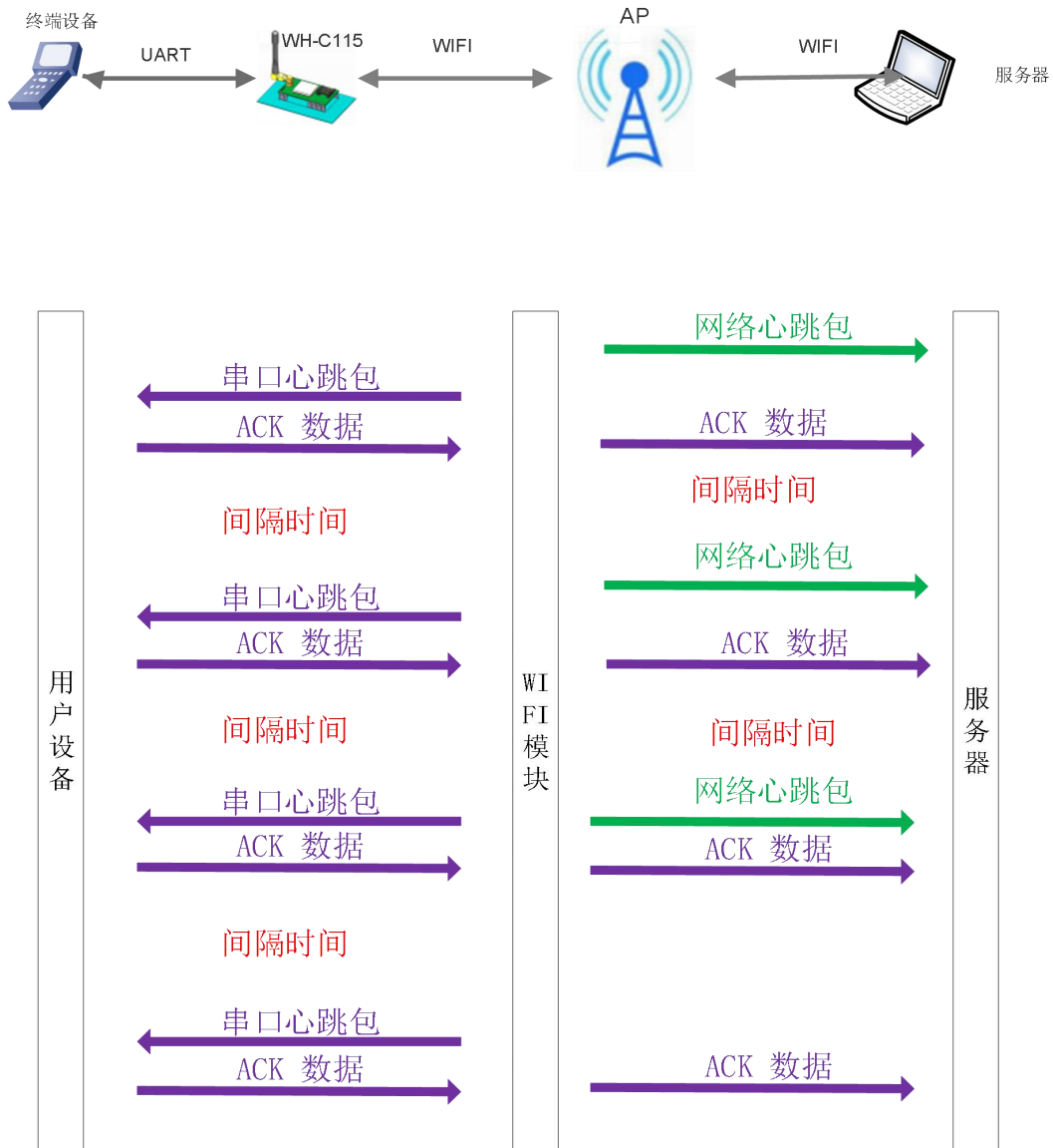
图 22 心跳包功能框图
