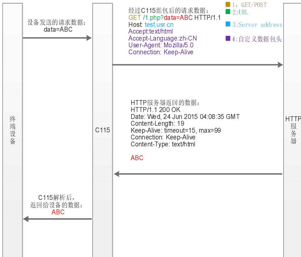
图 10 HTTPD Client 工作框图
