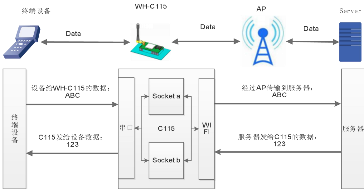
图 6 透明传输功能框图
