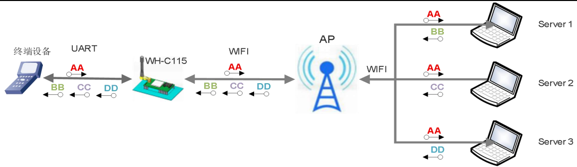
图 7 Socket 通信
