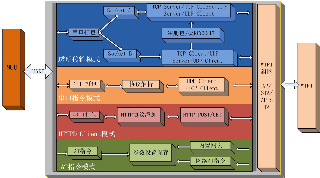
图 2 功能框图
