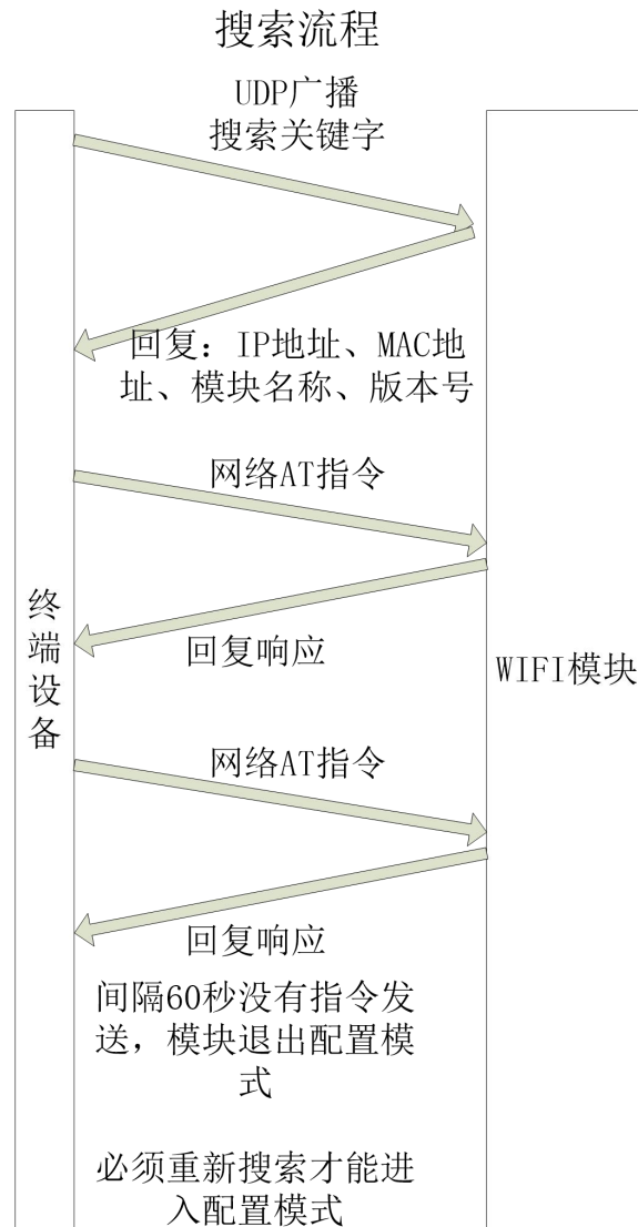
图 15 局域网搜索框图
