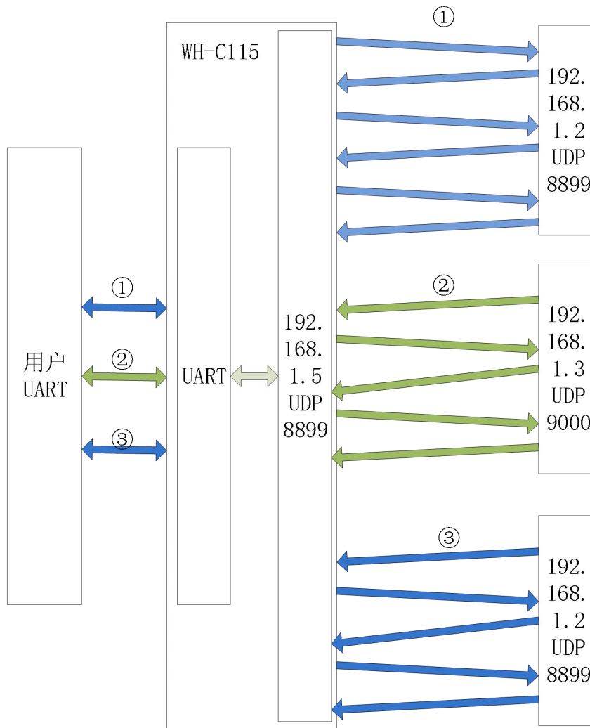
图 8 UDP Server 工作流程
