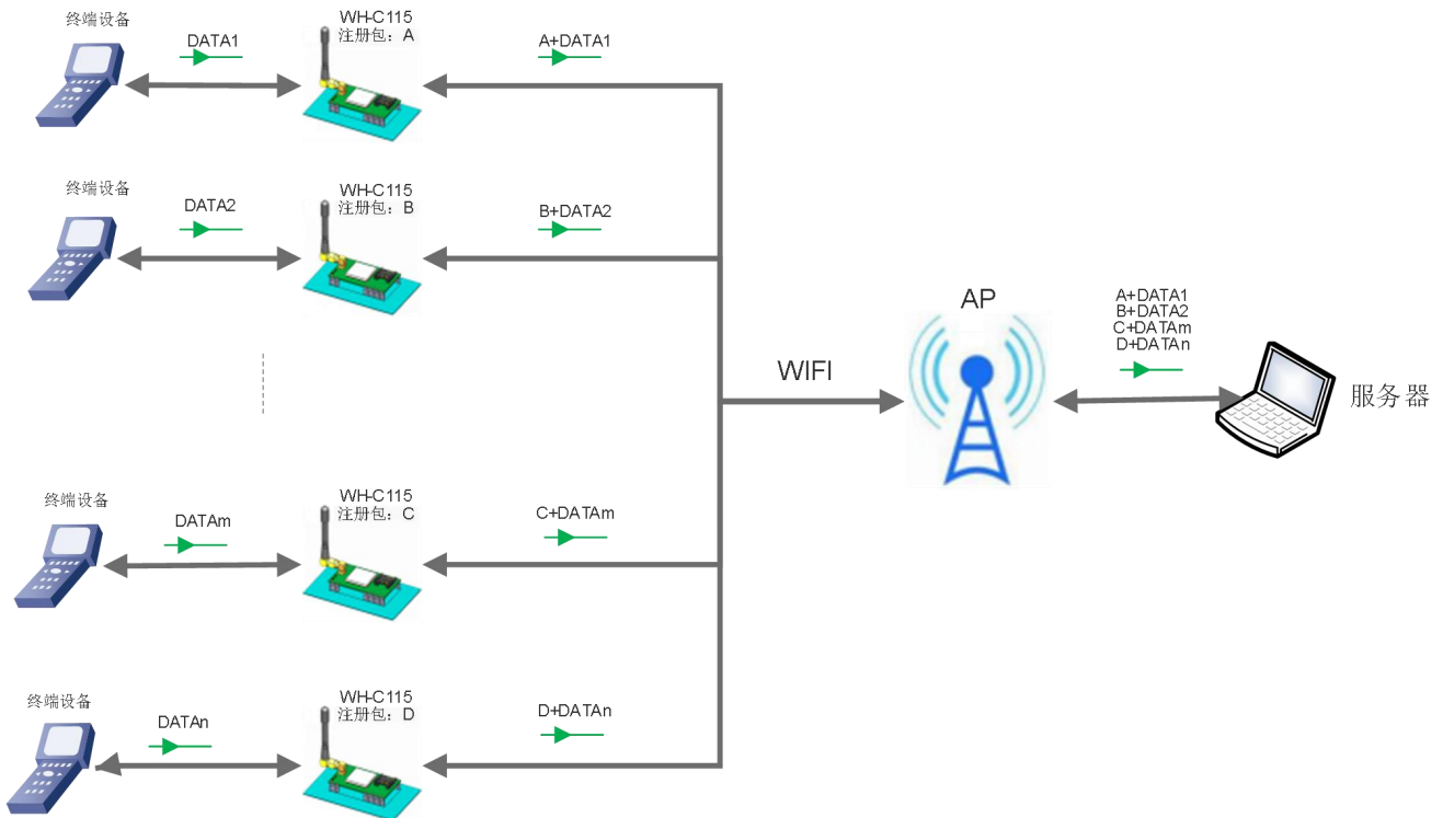
图 16 注册包功能框图
