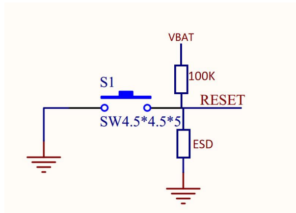
图片12 Reset 参考电路
