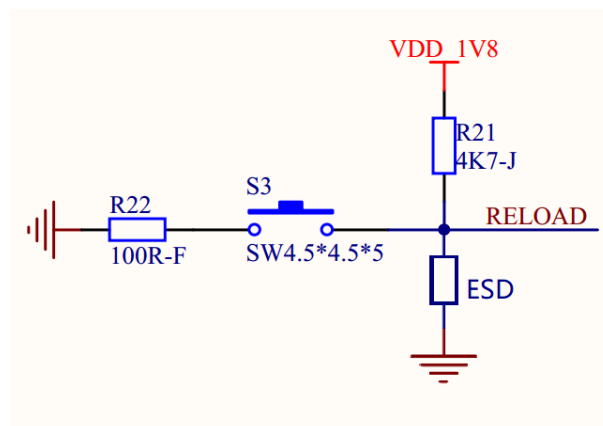
图片13 Reload 参考电路
