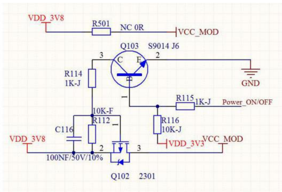
图片 5 模块电源控制参考电路
