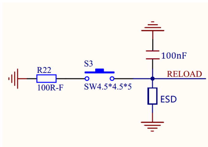
图片13 Reload 参考电路
