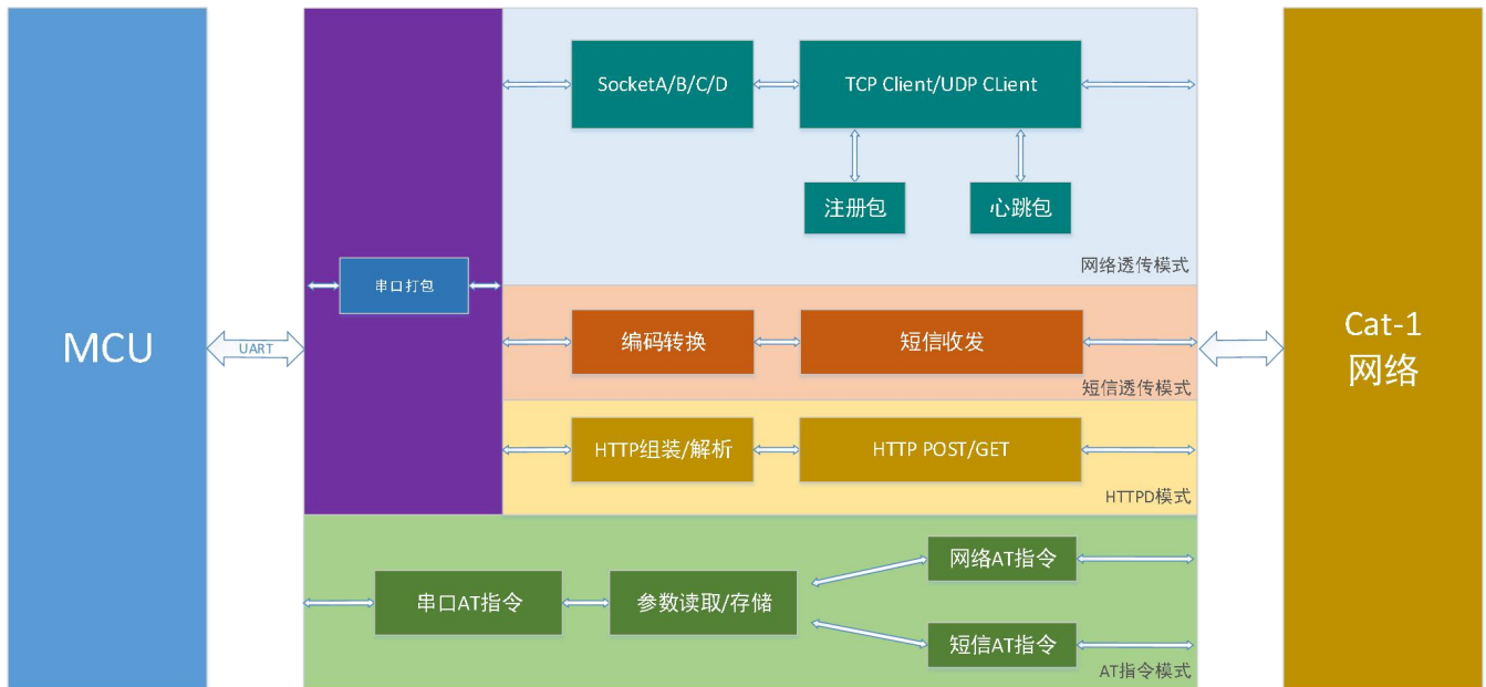
图 3. 功能框图
