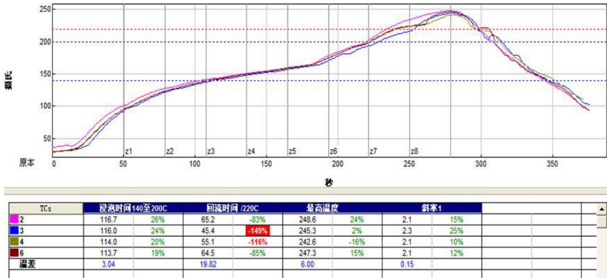
图片19 回流焊接温度曲线图
