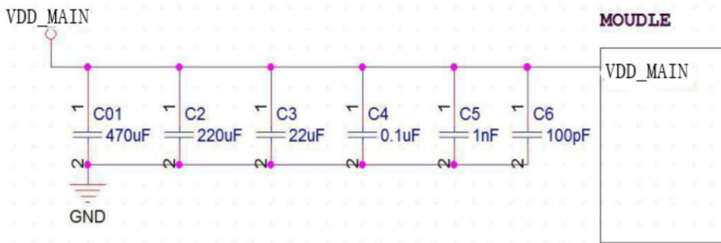
图片6 模块电源参考电路
