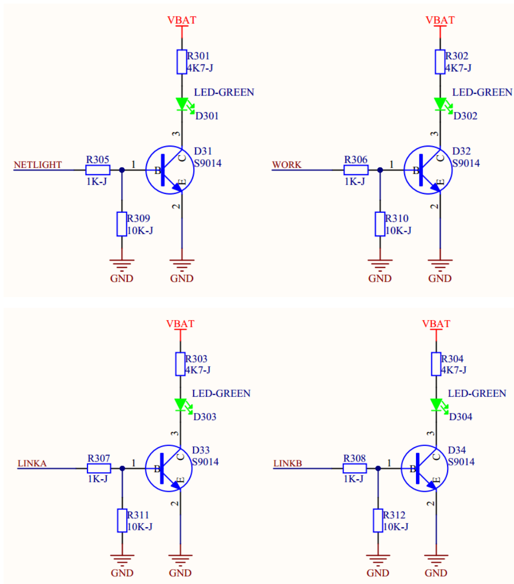
图片14 指示灯参考电路
