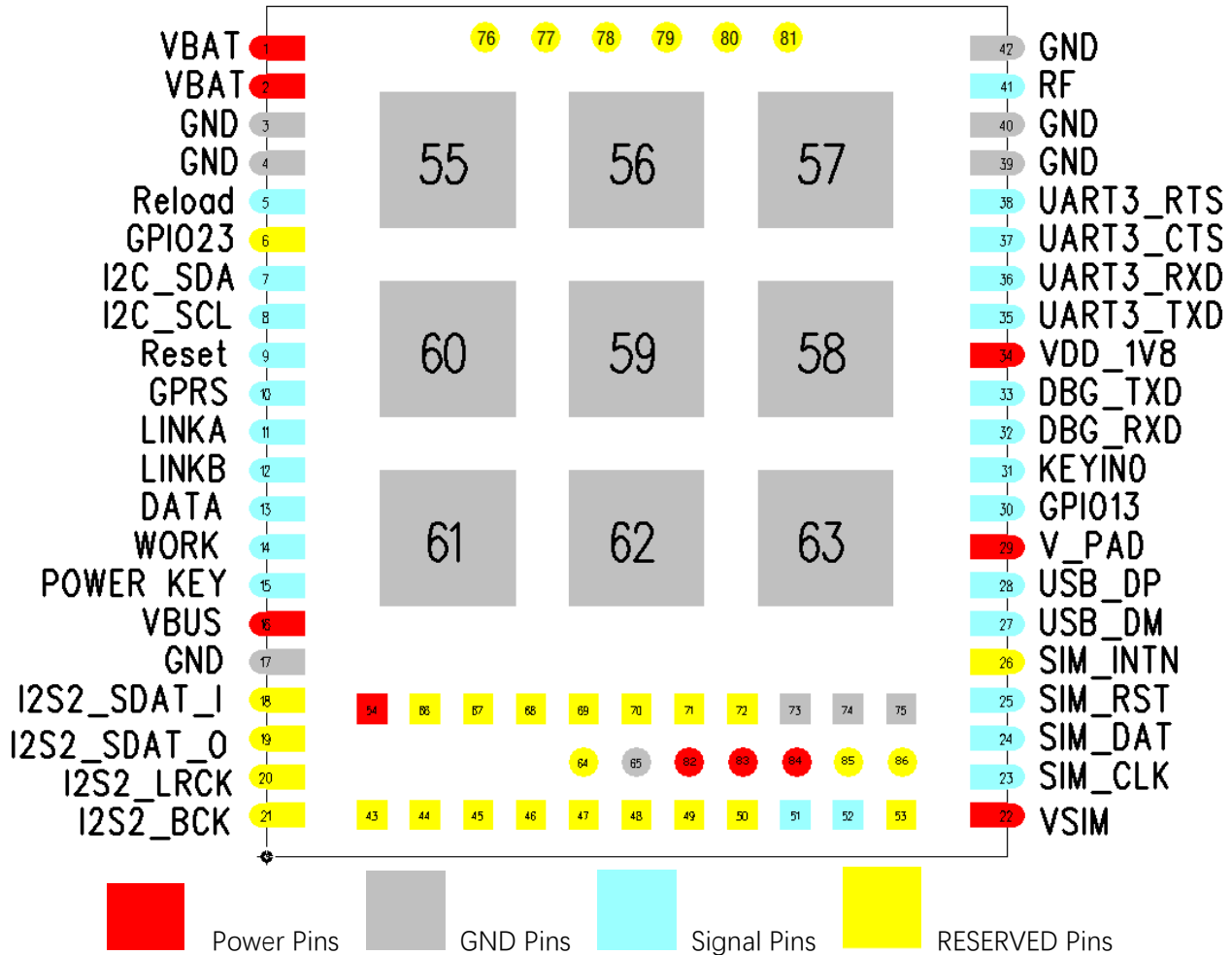
图片4 引脚标号 (TOP View)
