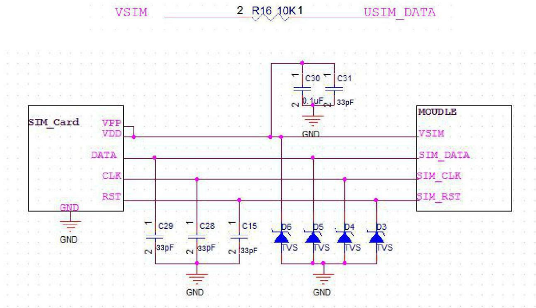
图片11 SIM 参考电路
