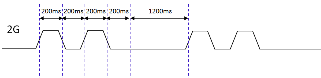
图片12 2G 网络连接指示
