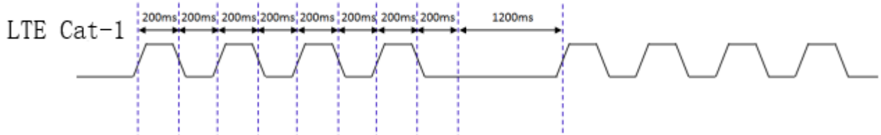
图片13 LTE Cat-1 网络连接指示
