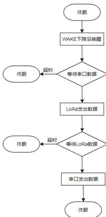
图 12 LSR 工作流程
