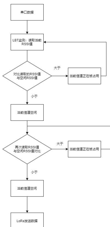
图 17 LBT 检测流程
