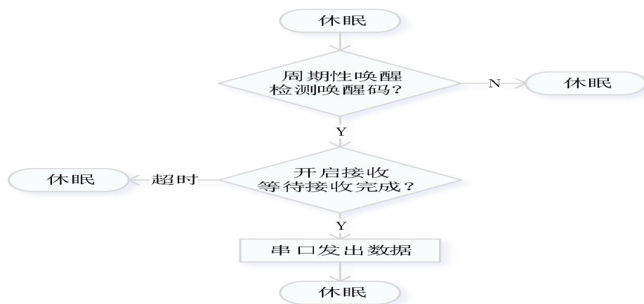
图 10 WU 和 LR 模式工作流程
