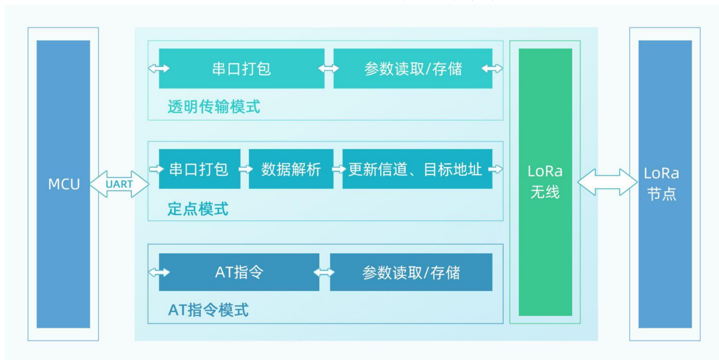
图 4 功能框图
