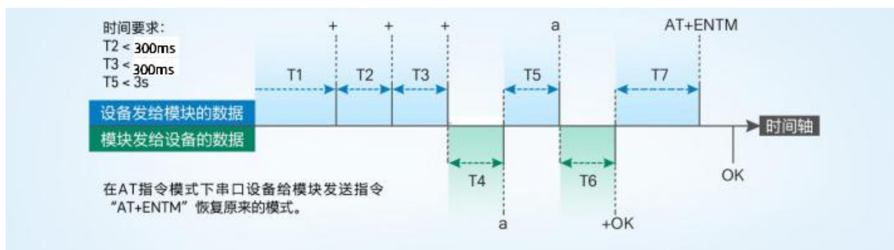
图 24 切换指令模式时序
