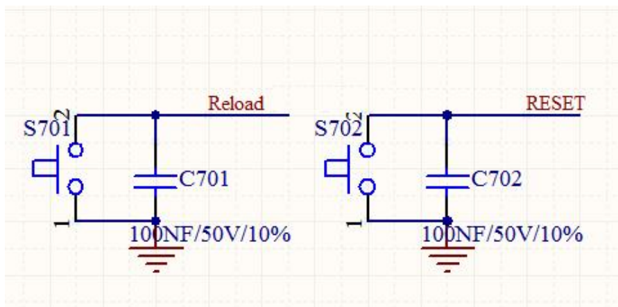
图片 11 Reload 和 Reset 按键控制电路图
