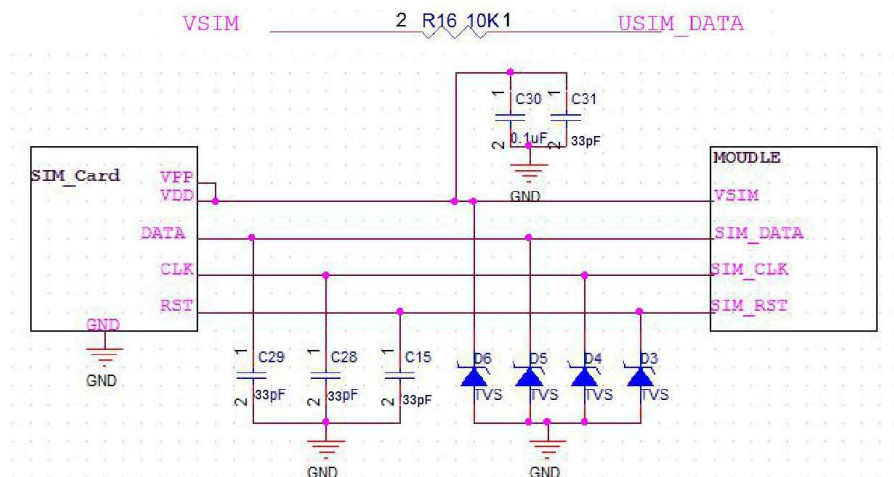
图片 8 SIM 卡参考电路
