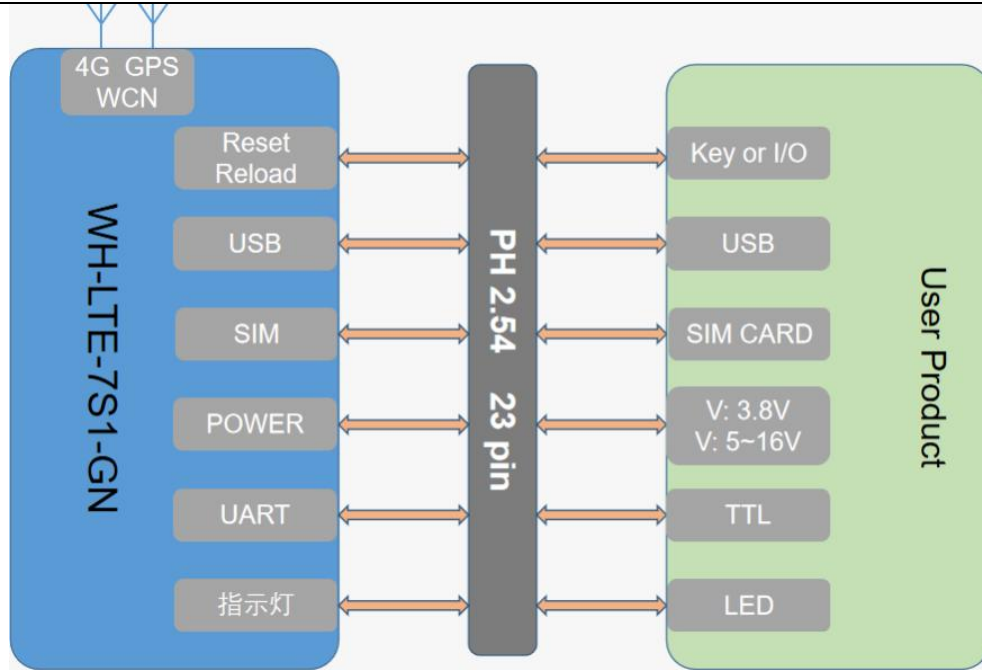
图片 1 模块应用框图
