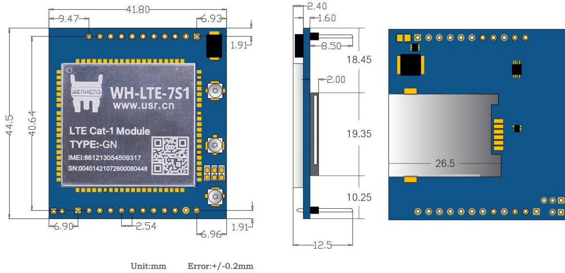
图片 10 WH-LTE-7S1-GN 尺寸说明
