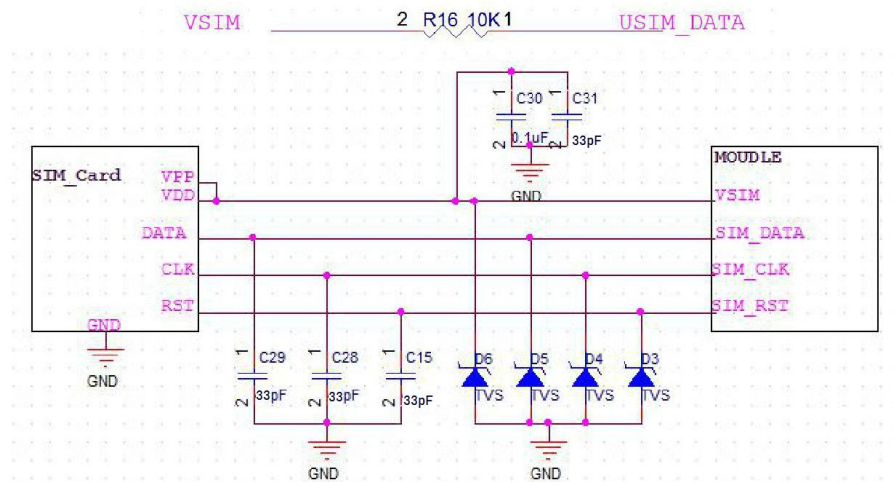
图片 6 SIM 卡参考电路
