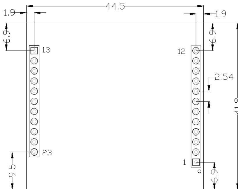
图片 11 USR-LTE-7S1-GN 推荐封装尺寸
