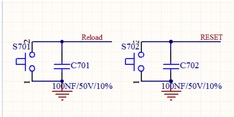
图片 8 Reload 和 Reset 设置控制电路图
