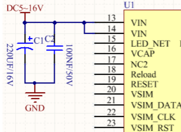
图片 3 模块电源参考电路
