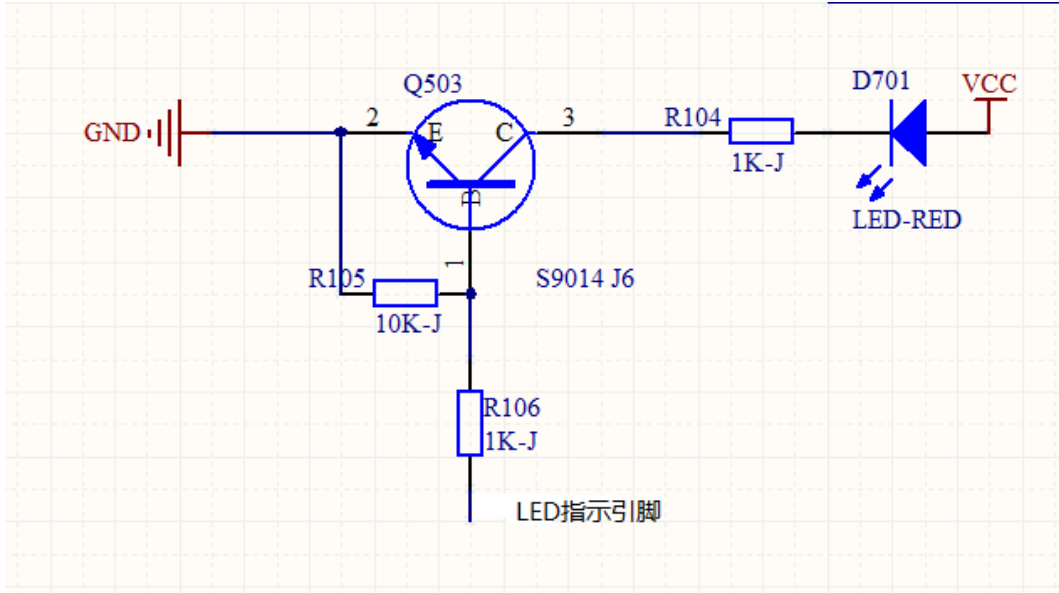
图片 7 指示灯参考电路
