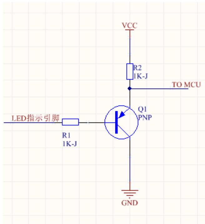
MCU 读取 LED 指示引脚参考电路
