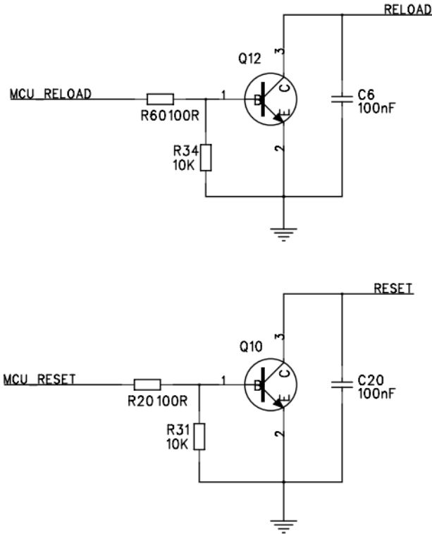
图片 10 Reload 和 Reset 用户 MCU 控制参考电路图
