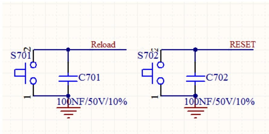
图片 9 Reload 和 Reset 按键控制电路图
