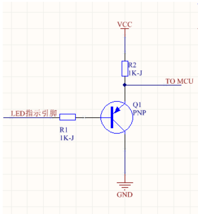
图片 8 MCU 读取 LED 指示引脚参考电路
