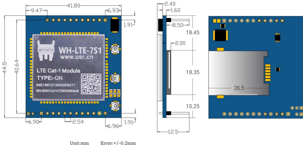
图片 12 WH-LTE-7S1-GN 尺寸说明
