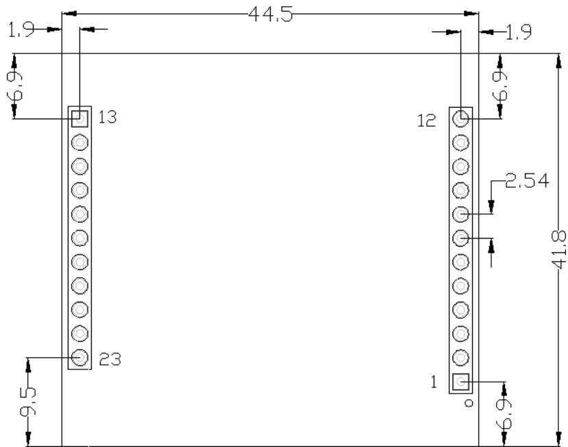
图片 13 USR-LTE-7S1-GN 推荐封装尺寸
