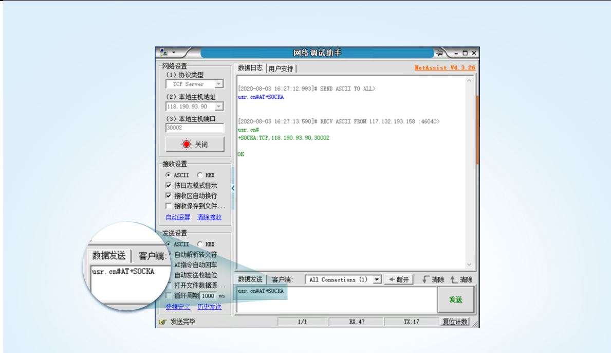
图35. 网络 AT 指令示意图
