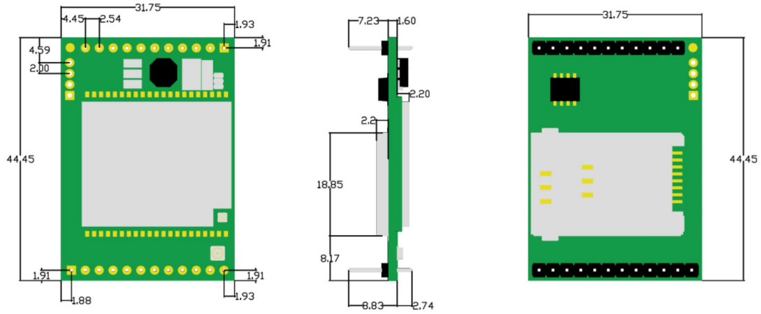
图6. WH-LTE-7S1 尺寸说明
