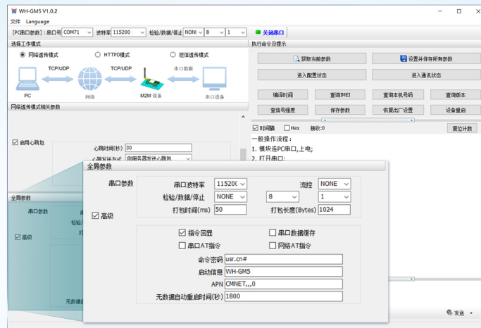
图31. 设置软件示意图
