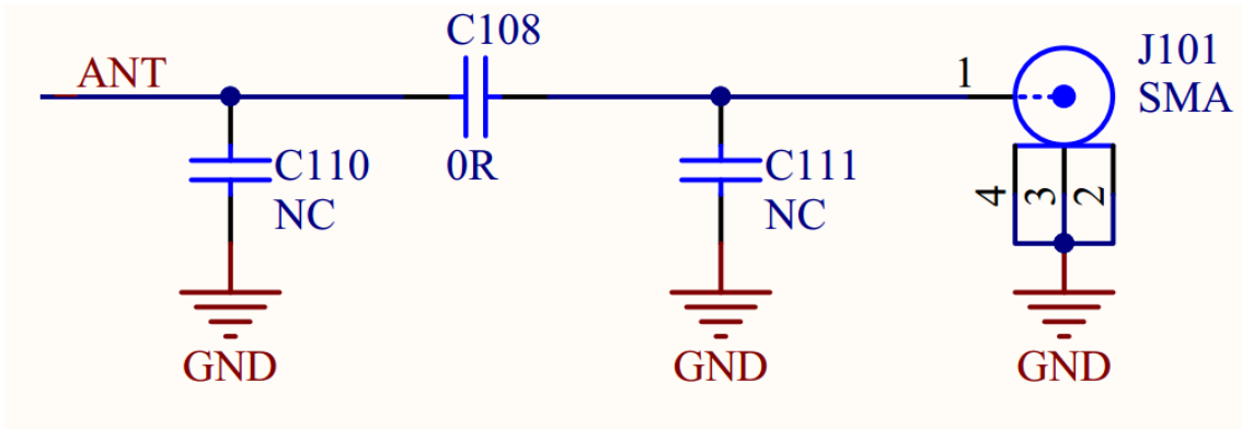
图片12 WH-NB61 预留匹配线路
