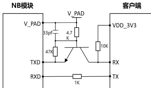
图片5 UART 电平转换参考设计
