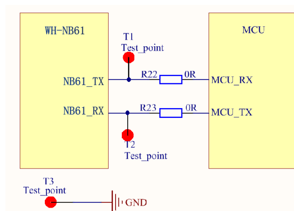
图片6 UART 预留测试点
