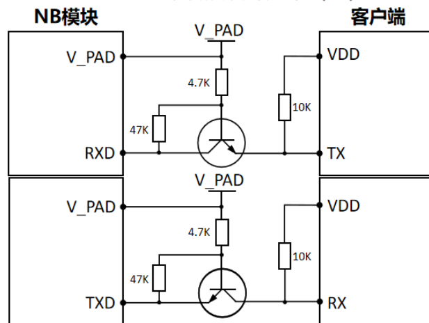
UART电平转换设计方案（一）
