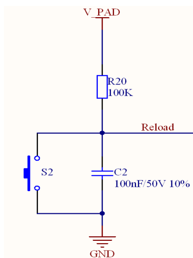
图片10 Reload 参考设计
