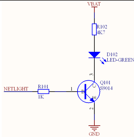
图片8 LED 参考设计
