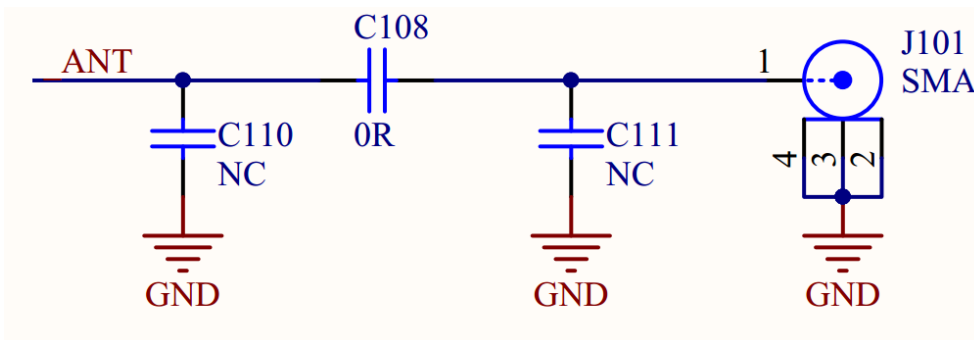
图片12 WH-NB63 预留匹配线路
