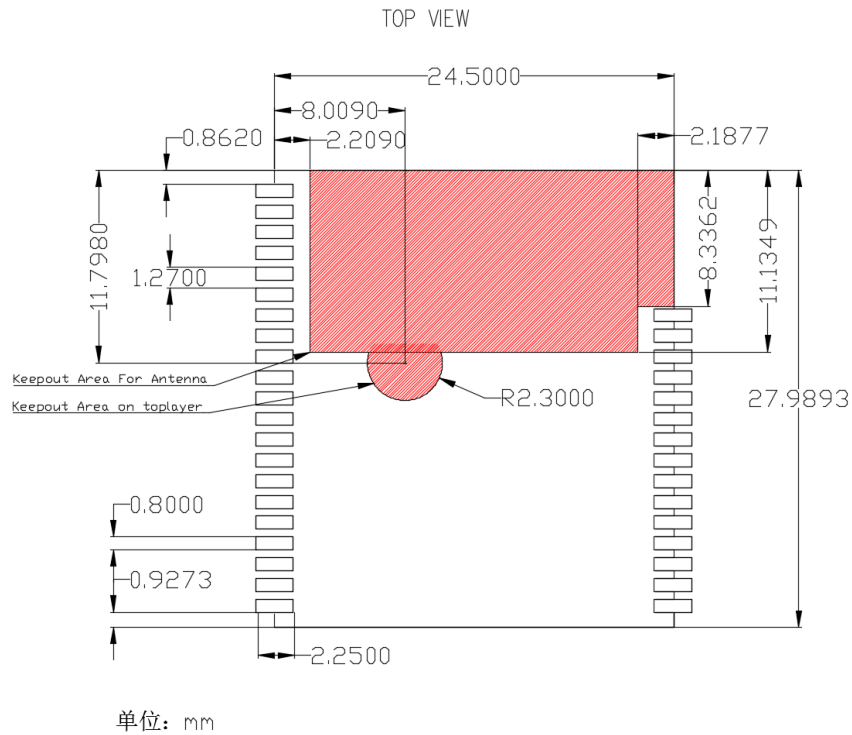
图片19 WH-NB63-BAA 内置天线模块 Layout 推荐封装尺寸
