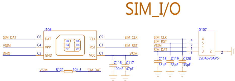
图片7 SIM 参考电路
