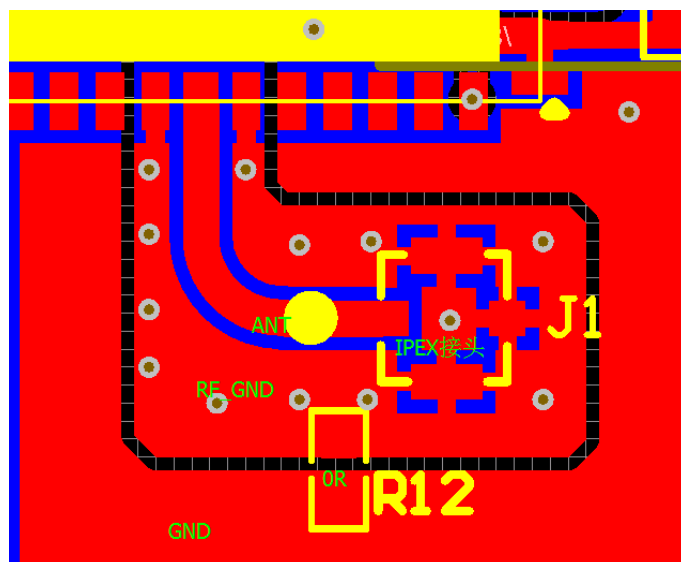
图片11 射频走线示意图
