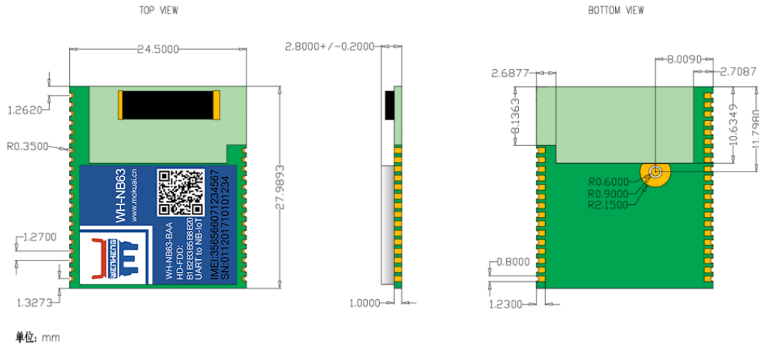
图片17 WH-NB63-BAA 内置天线模块尺寸说明
