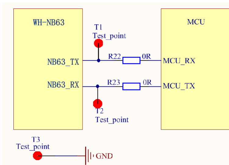
图片6 UART 预留测试点
