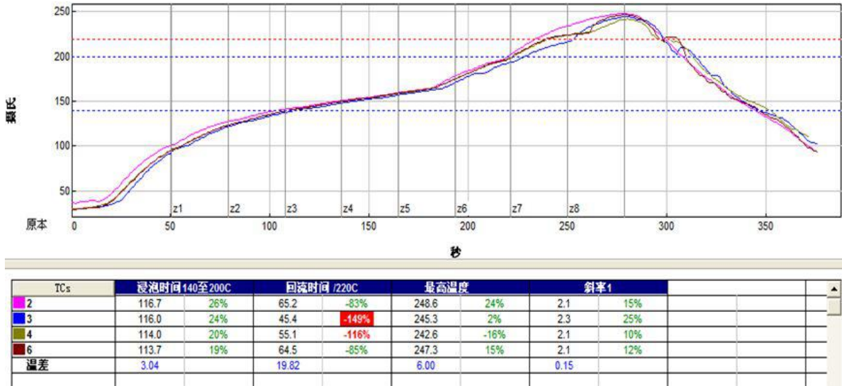
图片15 回流焊焊接温度曲线图
