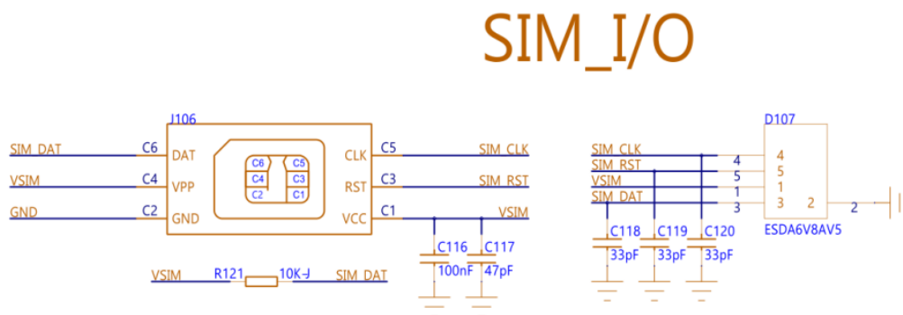
图片7 SIM 参考电路
