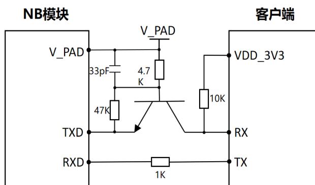
图片5 UART 电平转换参考设计
