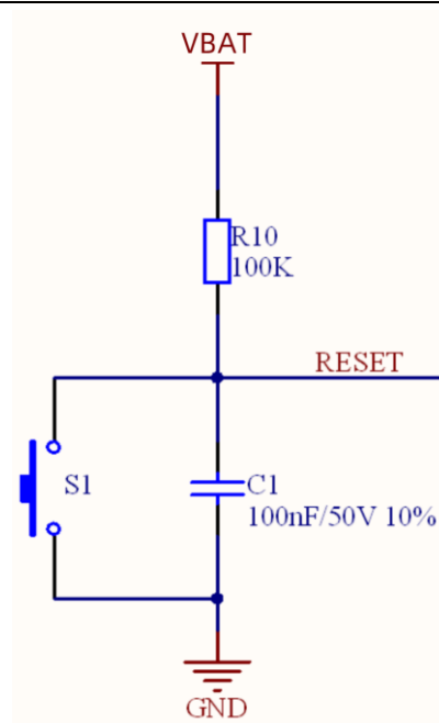
图片9 Reset 参考设计
