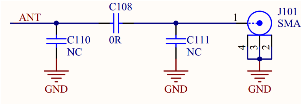
图片12 WH-NB63 预留匹配线路
