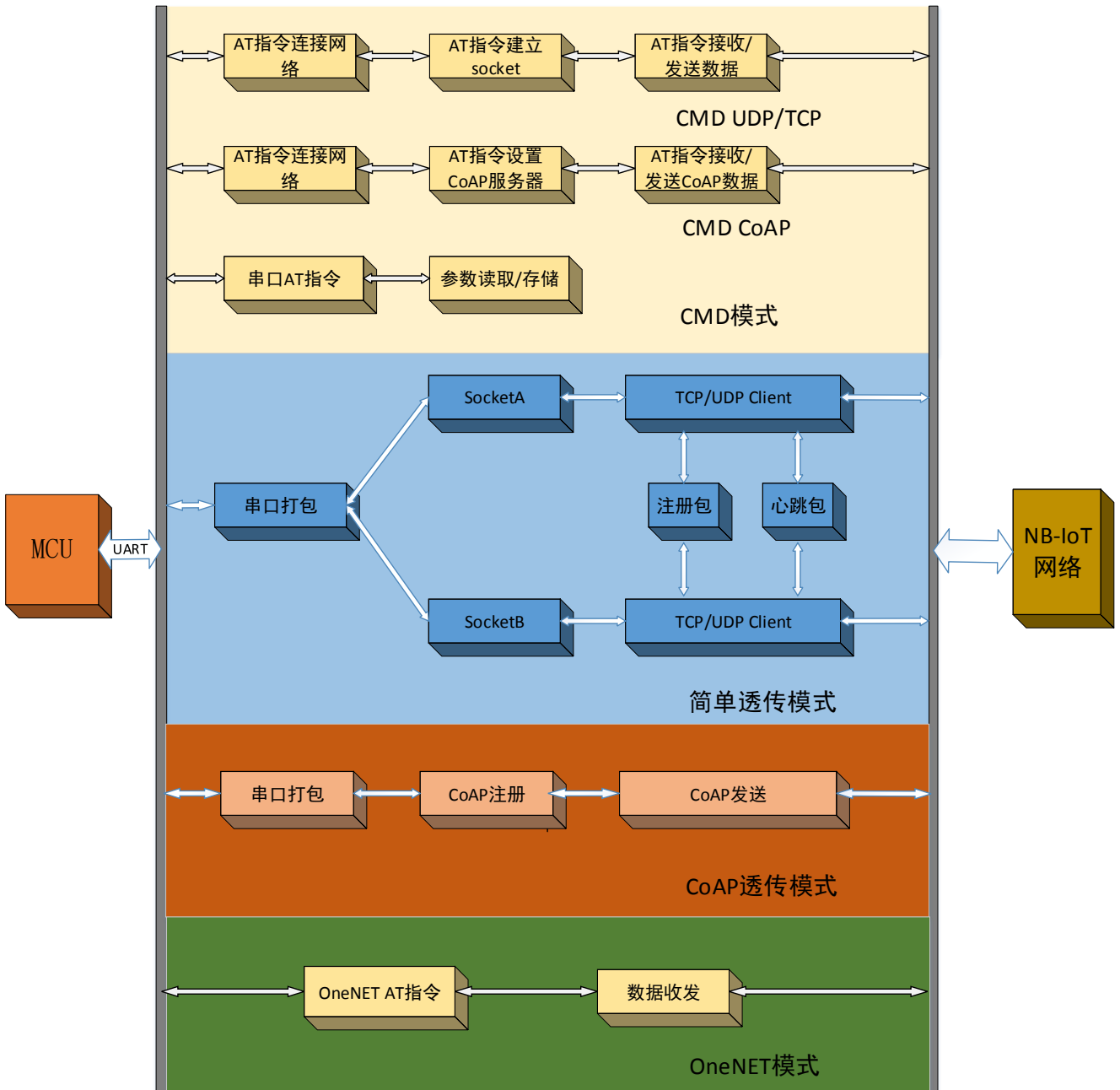
图 1 工作模式结构图
