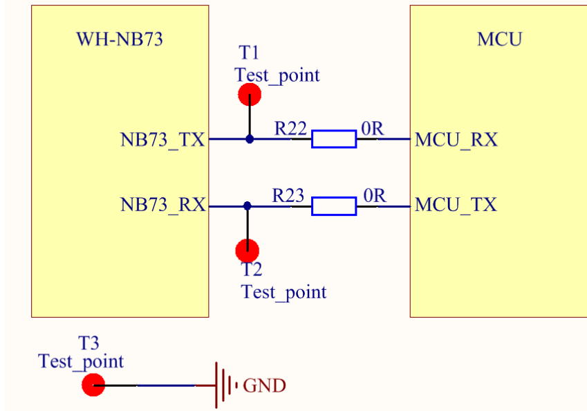
图片6 UART 预留接口
