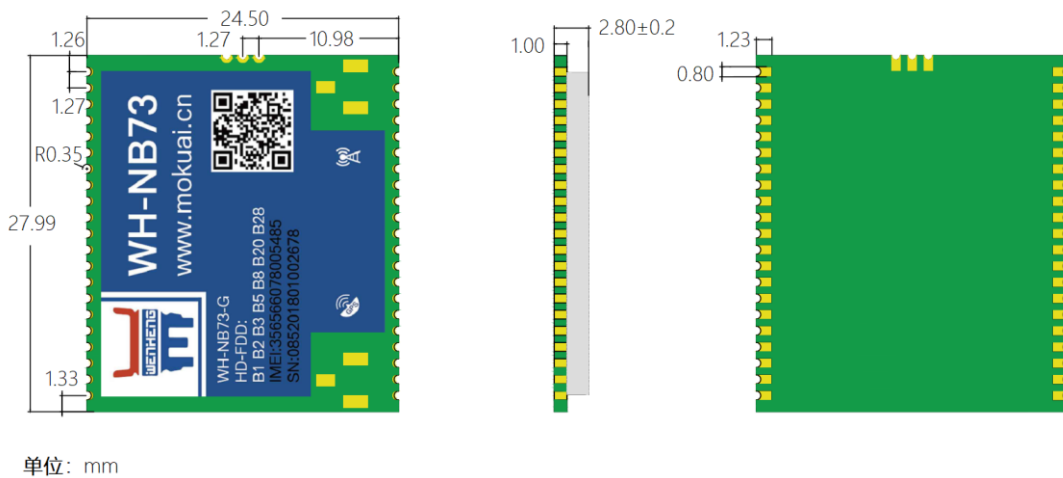
图片16 WH-NB73-G 尺寸说明
